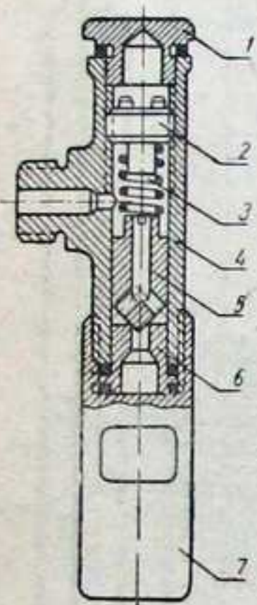
Фиг. 60. Редуктор-автомат.
