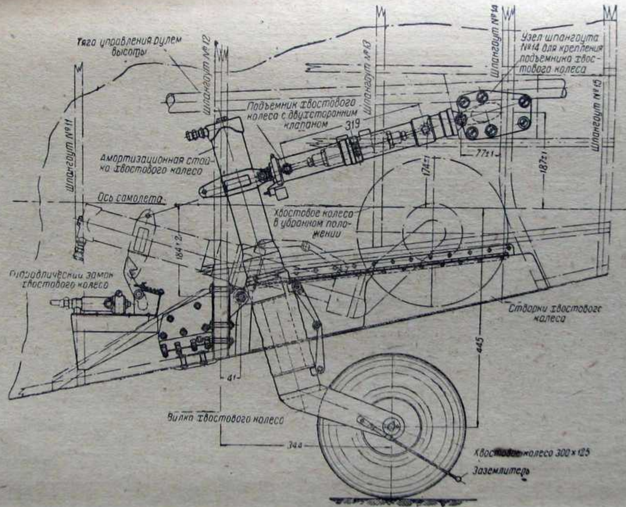
Фиг. 35. Установка хвостового колеса.
