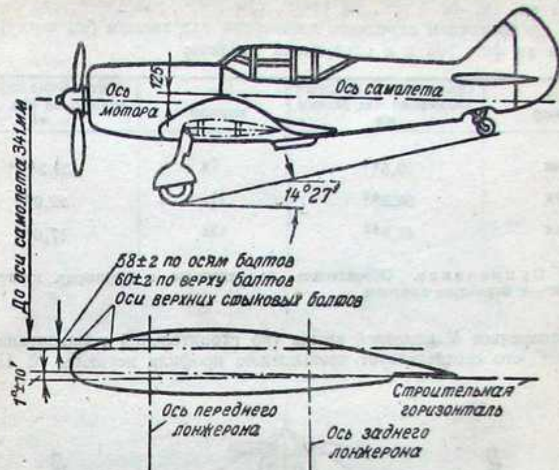
Фиг. 102. Установка самолета в линию полета.
