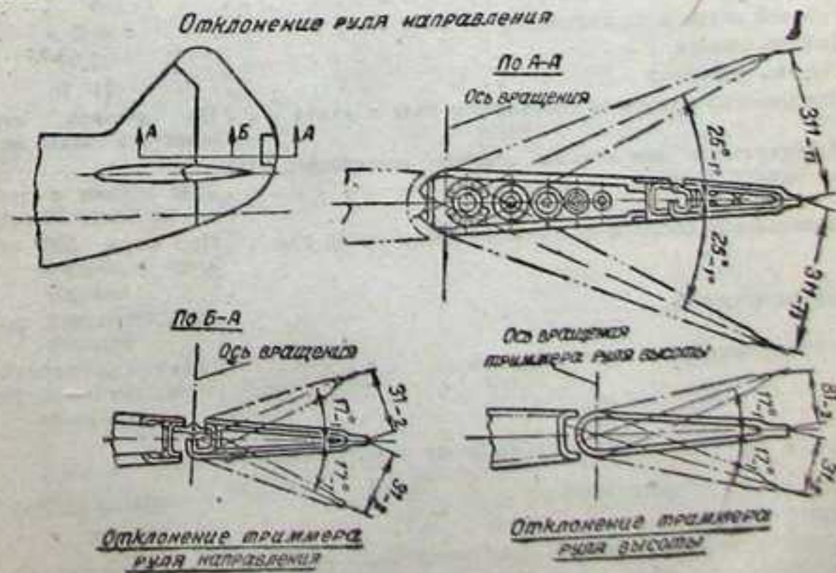
Фиг. 110. Отклонения руля направления и триммеров.
