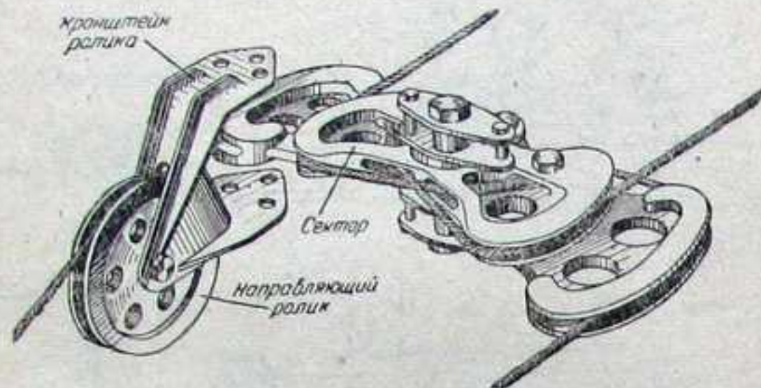
Фиг. 92. Сектор ножного управления.
