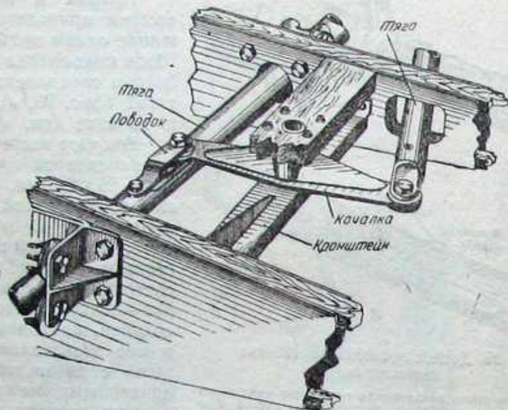
Фиг. 101. Качалка управления закрылками.
