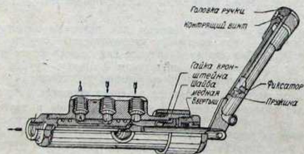
Фиг. 62. Распределительный кран закрылков (обозначения те же, что и на фиг. 61).
