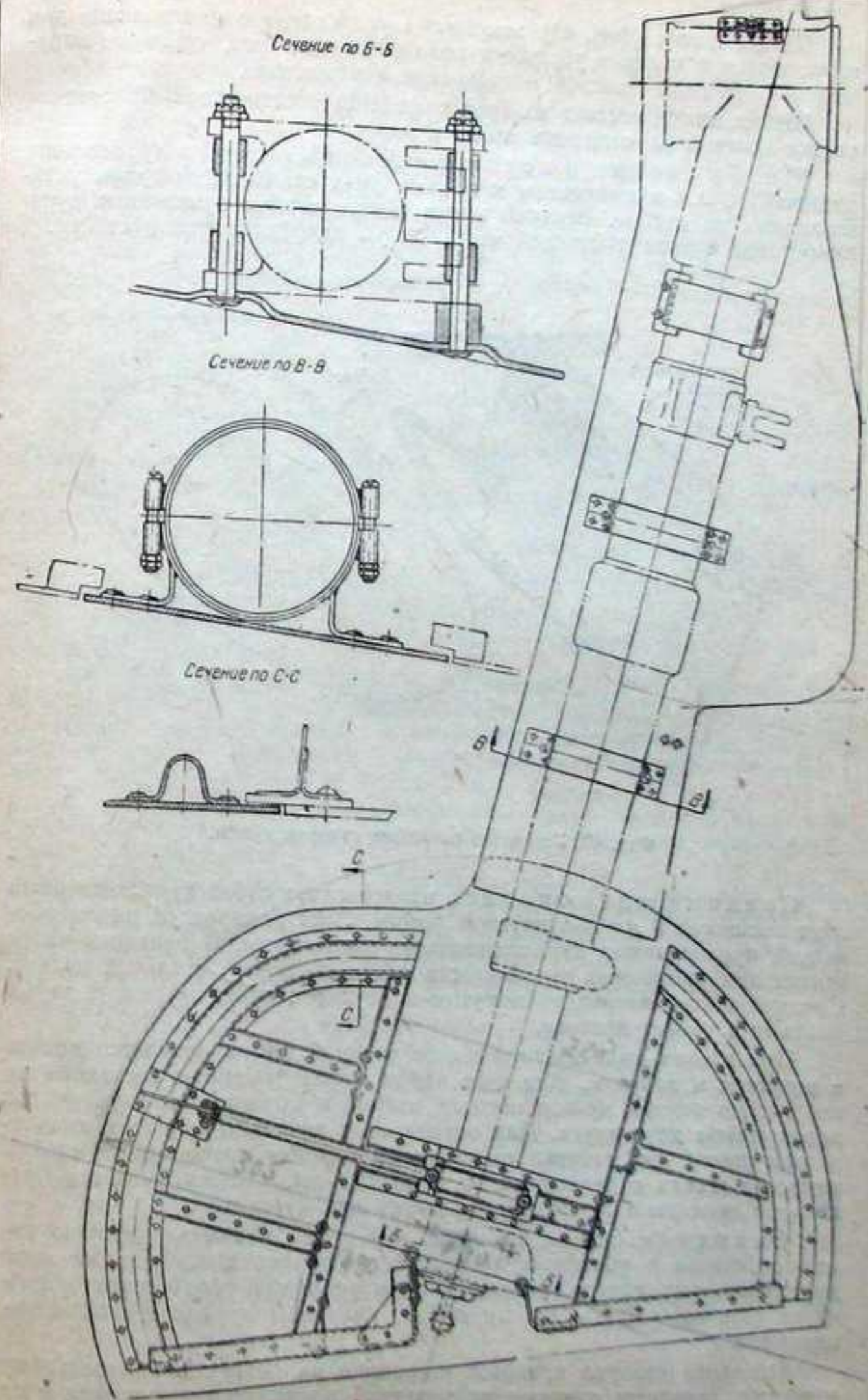
Фиг. 48. Щиток шасси.
