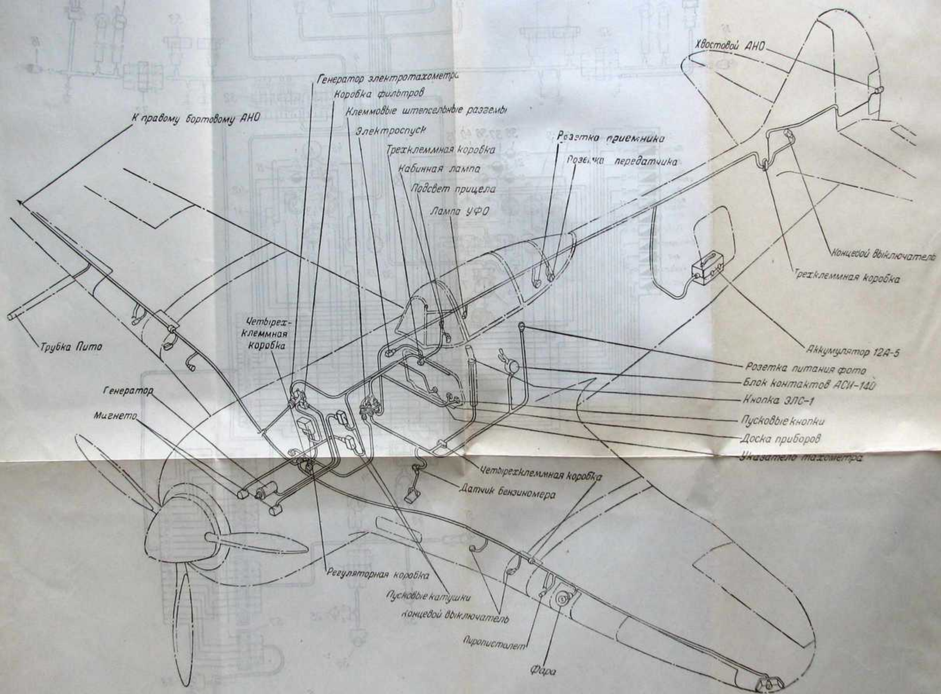
Фиг. 160. Схема расположения электроагрегатов на самолете.
