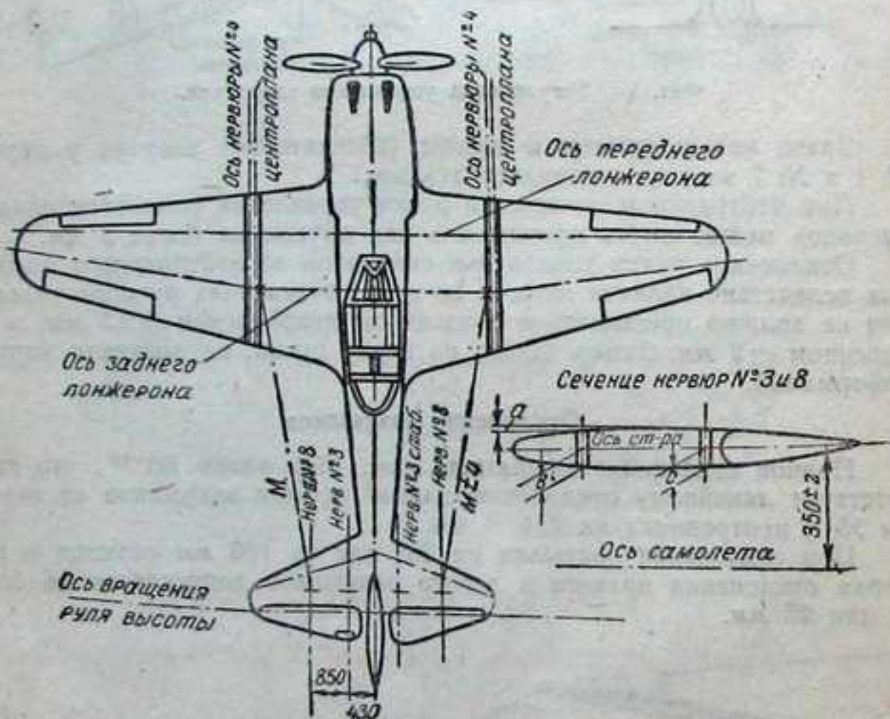
Фиг. 108. Установка и регулировка стабилизатора.
