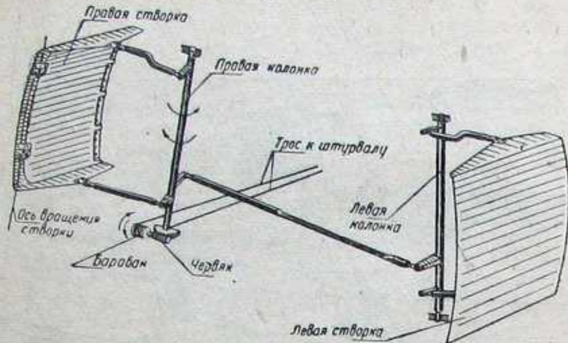
Фиг. 140. Схема управления боковыми створками.
