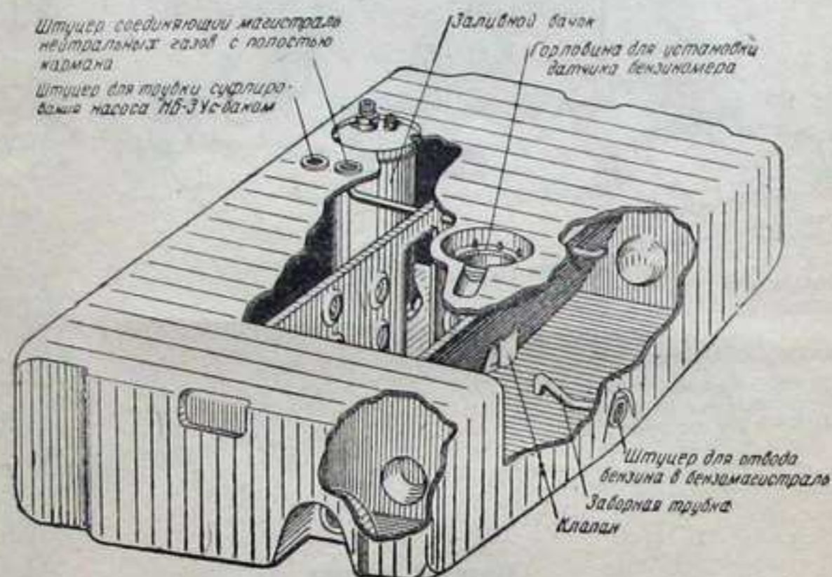
Фиг. 120. Бензобак.
