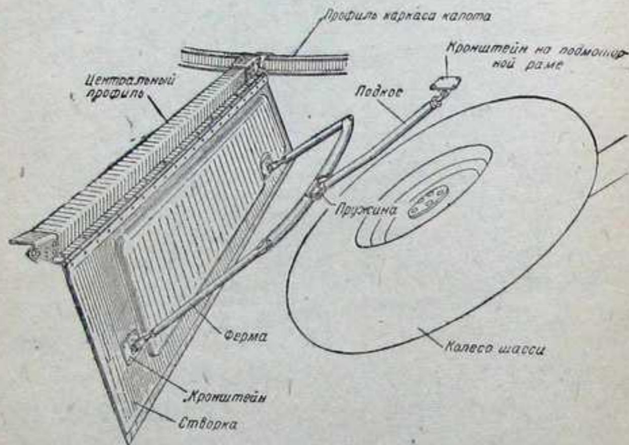
Фиг. 49. Установка откидных створок шасси.
