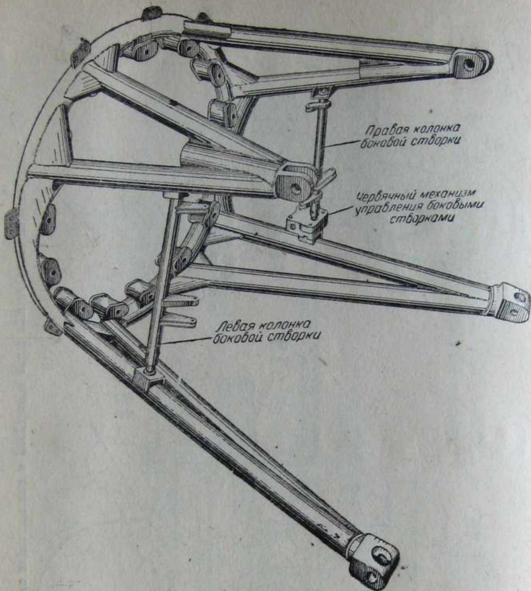
Фиг. 112. Моторная рама
