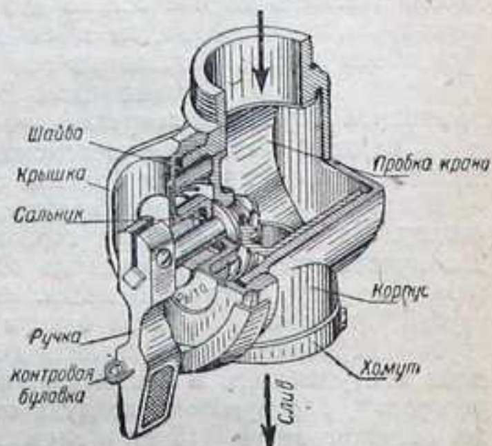
Фиг. 133. Сливной кран маслосистемы.
