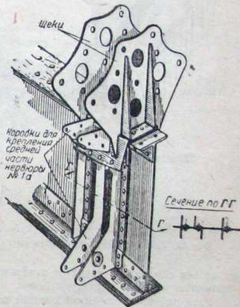
Фиг. 17. Задний узел крепления центроплана к фюзеляжу.
