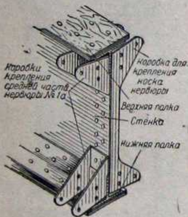
Фиг. 15. Типовое крепление нервюры к лонжерону центроплана.
