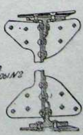
Фиг. 22. Передний лонжерон консоли крыла.
