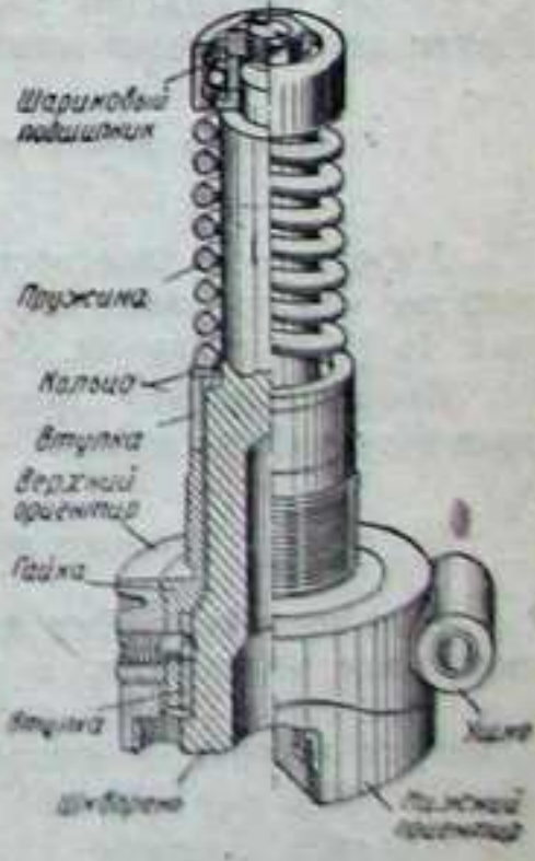
Фиг. 52. Ориентир хвостового колеса.
