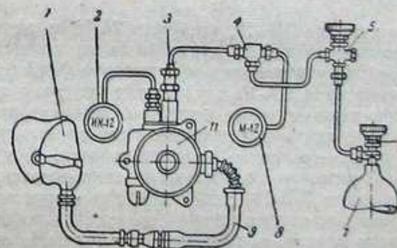
Фиг. 146. Принципиальная схема кислородного прибора КП-12.
