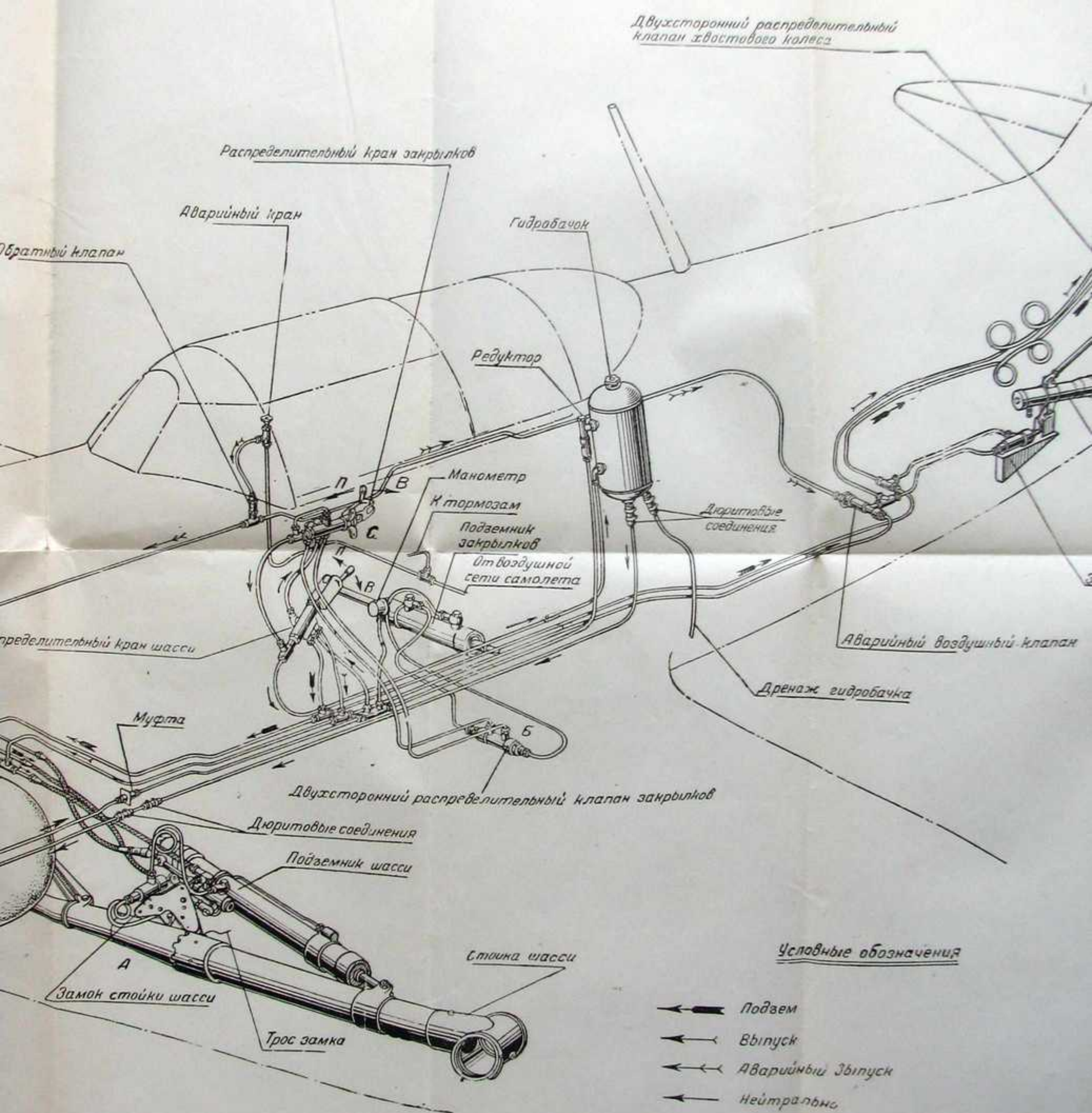
Фиг. 36. Гидросистема самолета.
