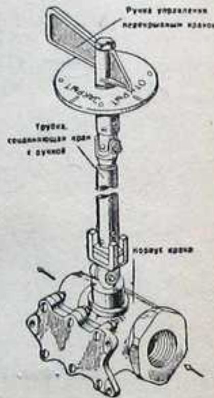
Фиг. 125. Перекрывной бензокран.
