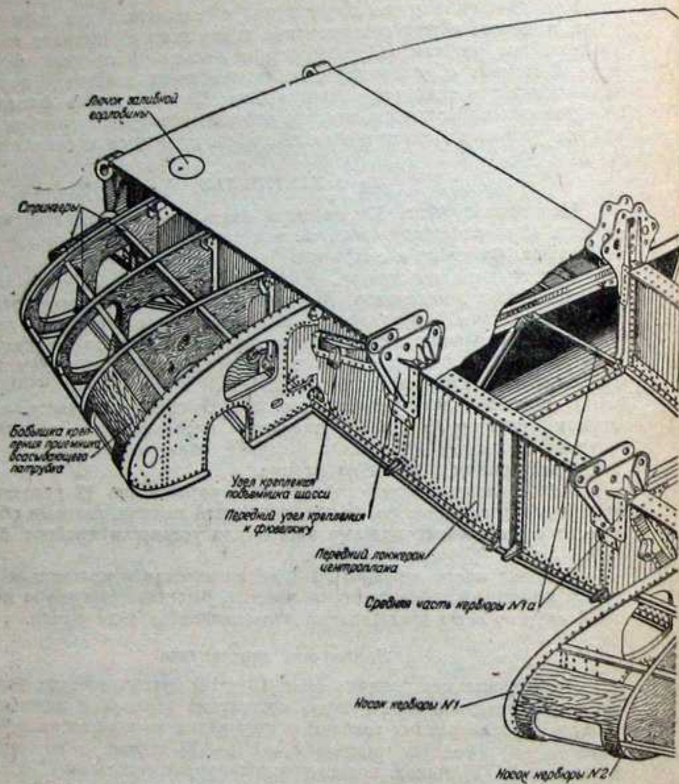
Фиг. 12. Центроплан.
