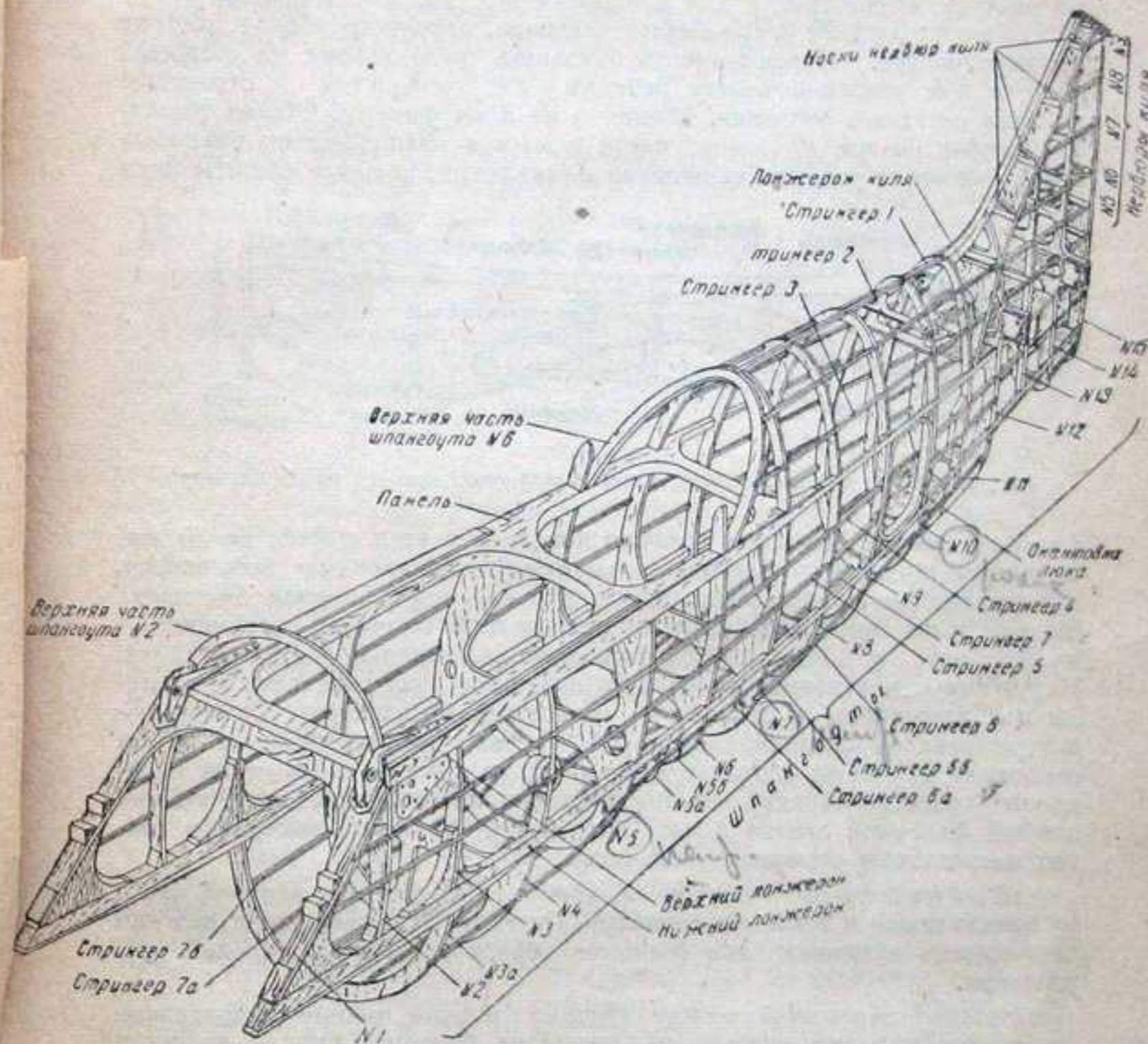
Фиг. 5. Каркас фюзеляжа.
