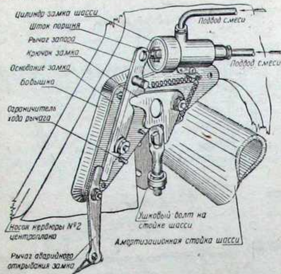
Фиг. 46. Замок шасси.
