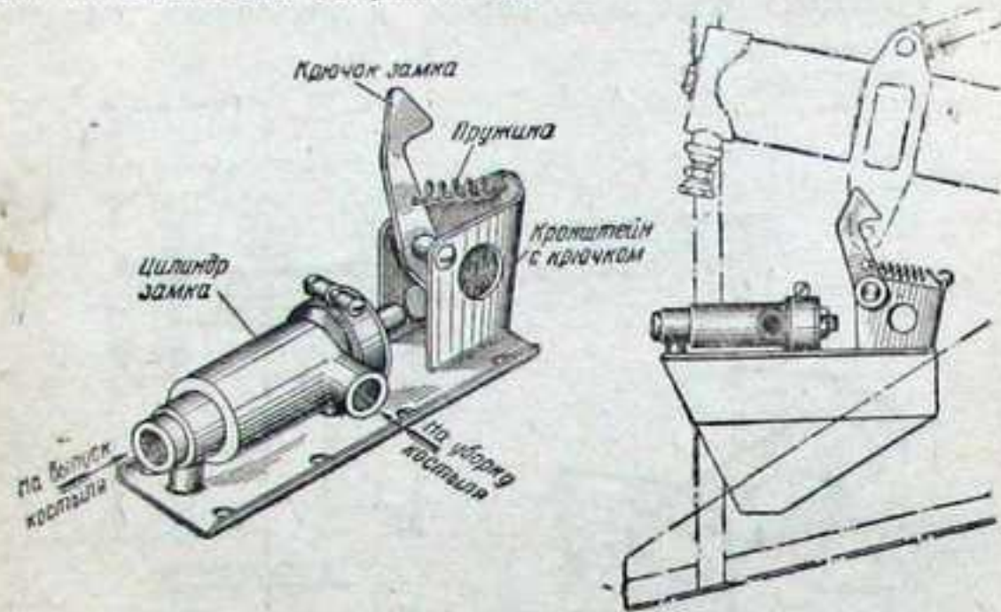
Фиг. 56. Замок хвостового колеса.
