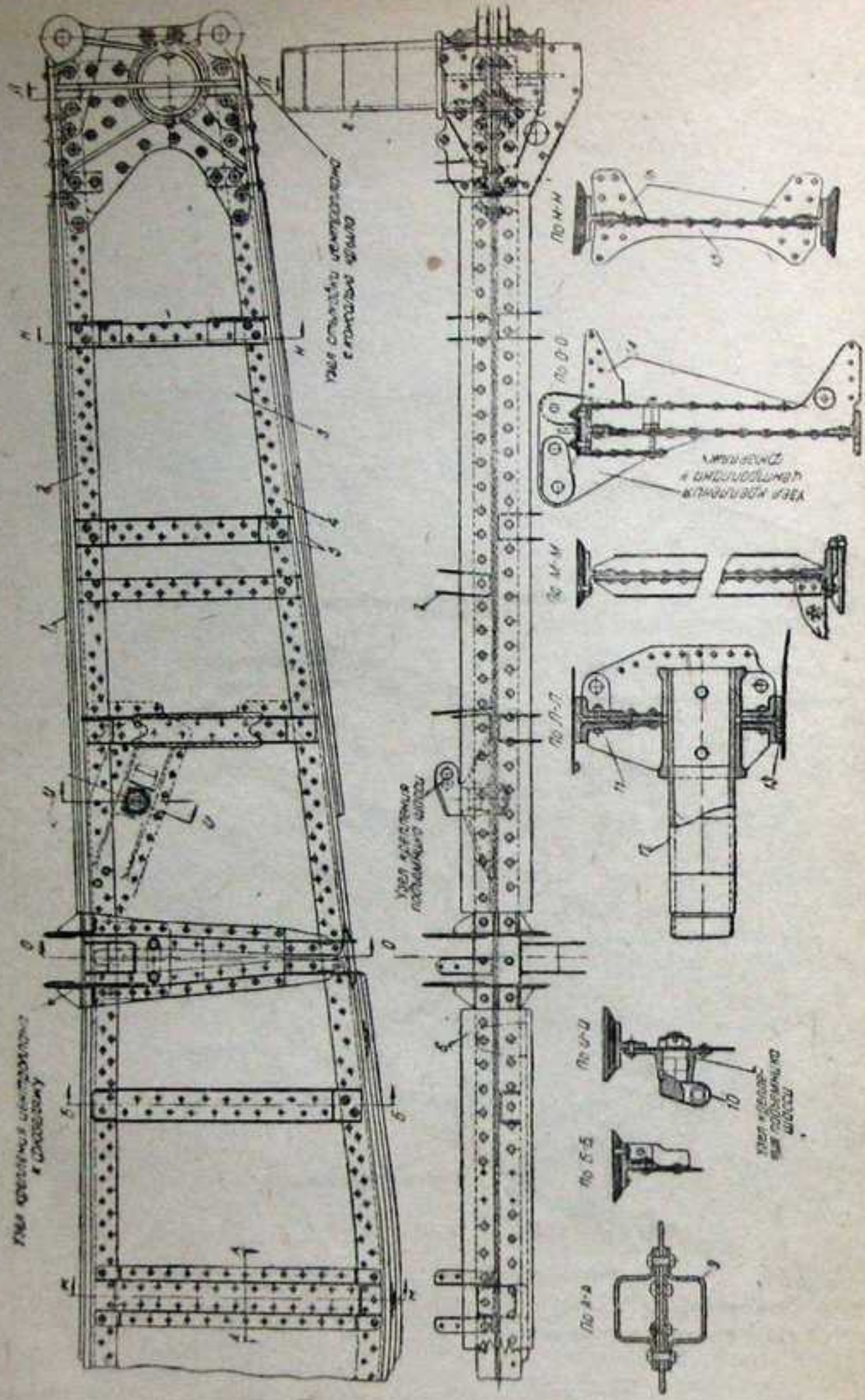
Фиг. 13. Передний лонжерон центропалки.
