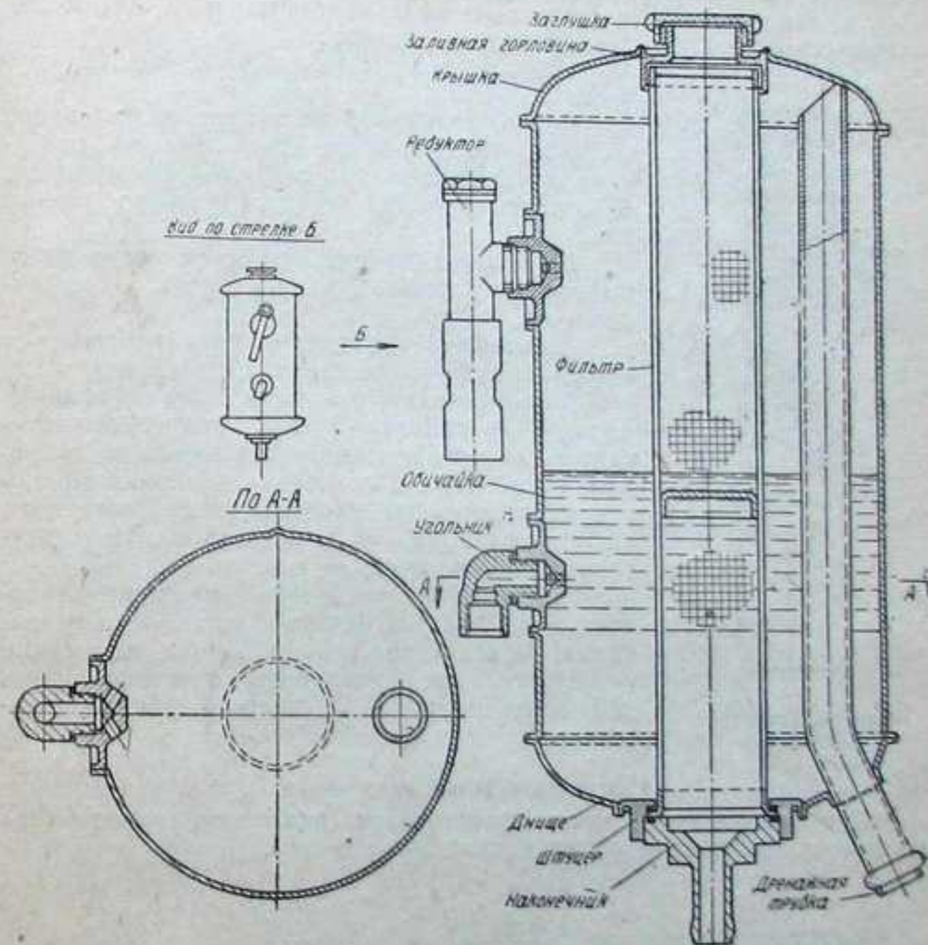
Фиг. 59. Гидробачок.
