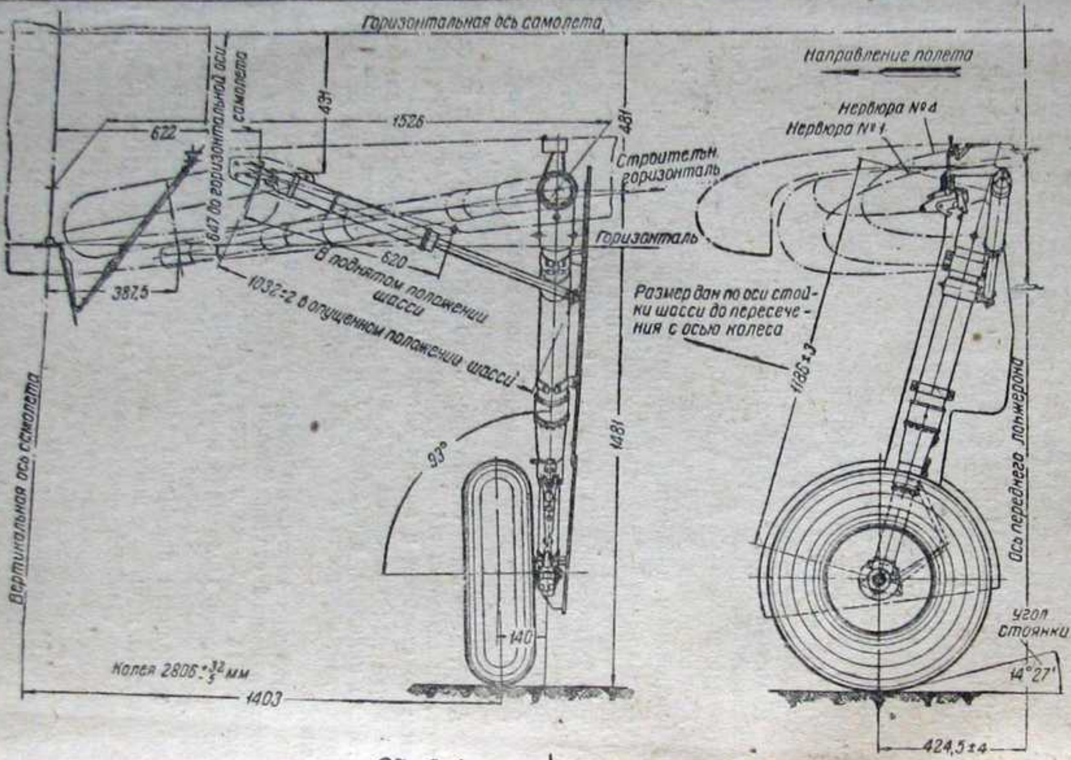
Фиг. 34. Установка шасси.
