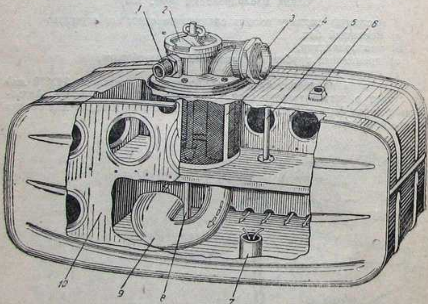
Фиг. 131. Масляный бак.
