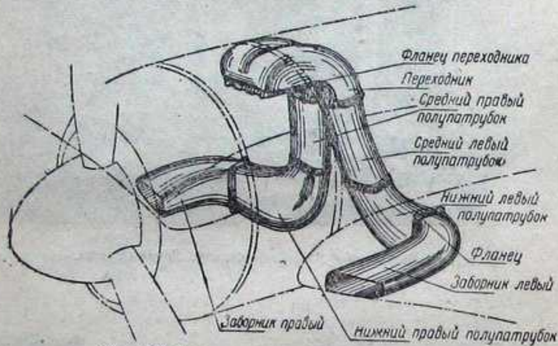
Фиг. 136. Всасывающие патрубки нагнетателя.
