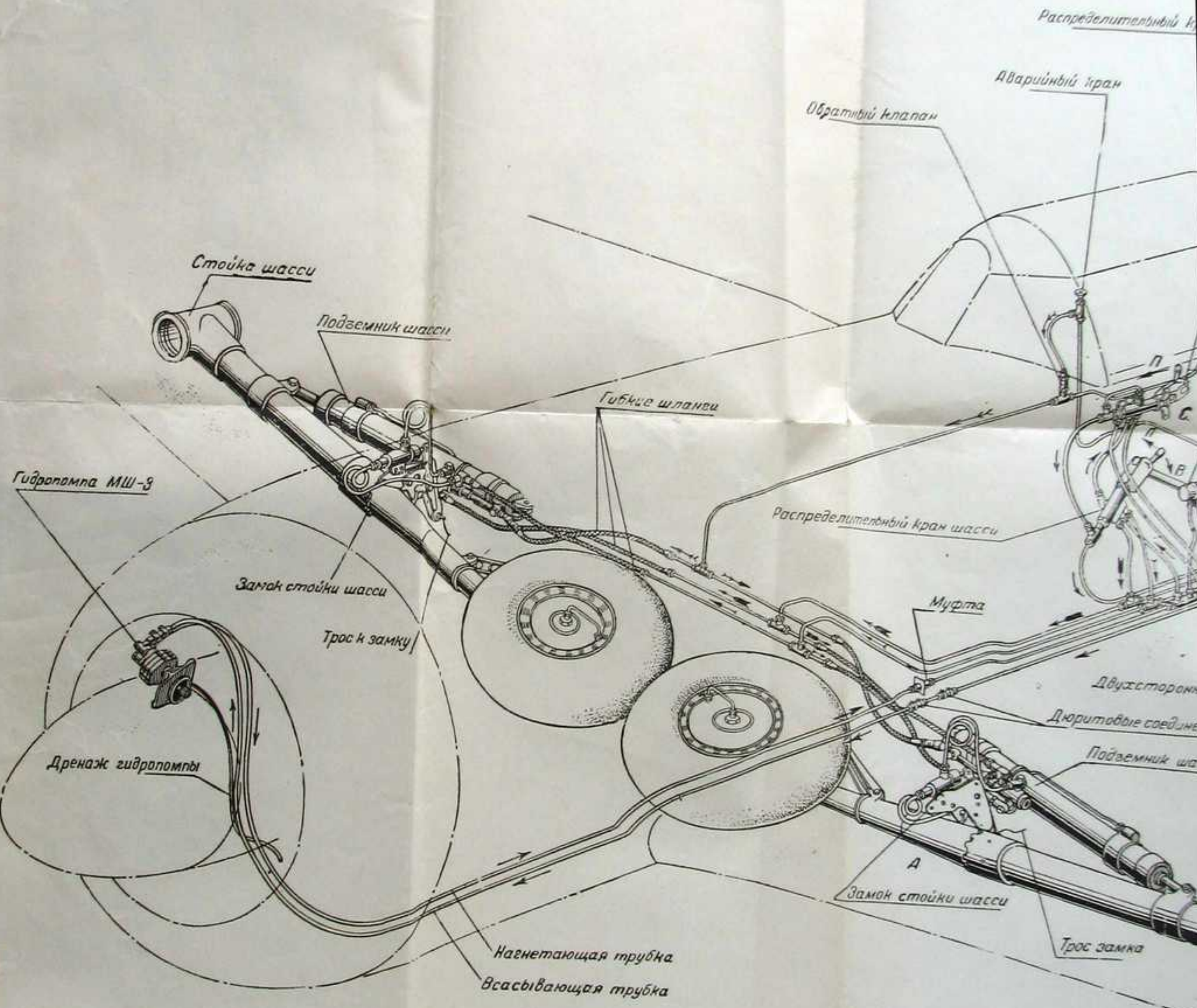
Фиг. 36. Гидросистема
