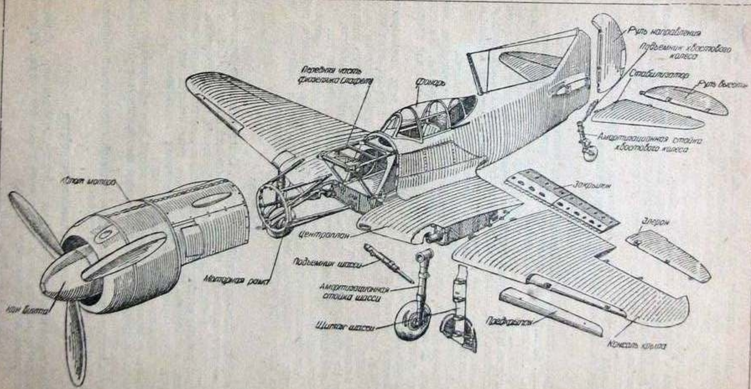
Фиг. 2. Схема разбега самолета на основные агрегаты.
