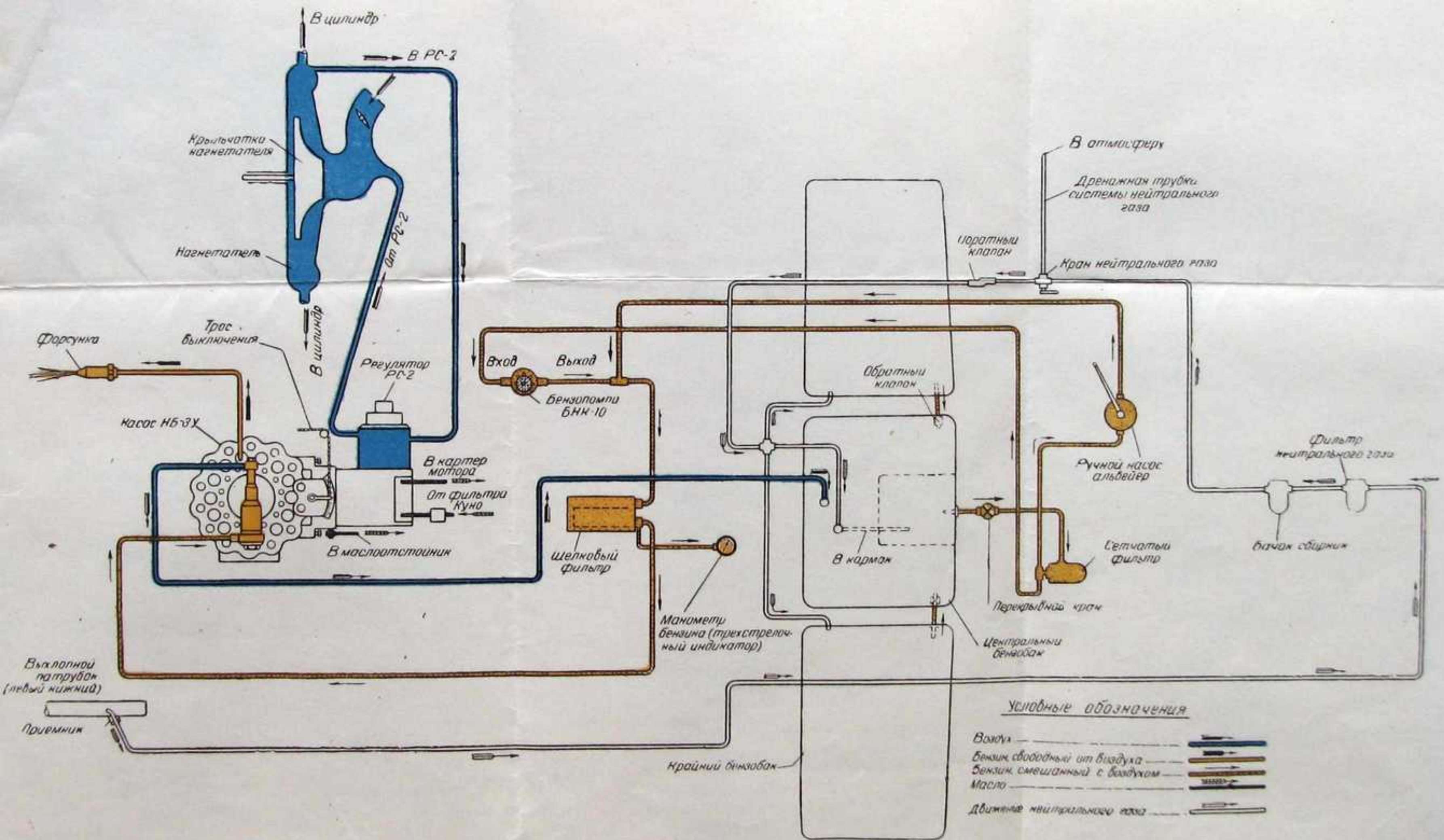
Фиг. 119. Принципиальная схема бензосистемы.
