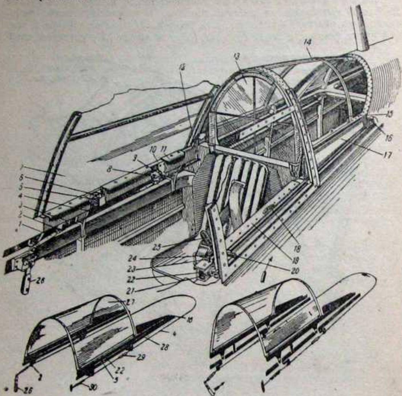
Фиг. 11. Фонарь самолета.
