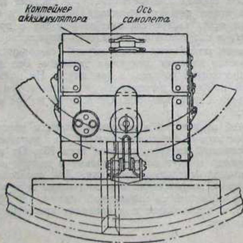
Фиг. 151. Установка контейнера аккумулятора.
