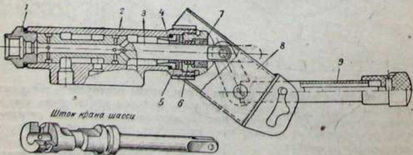
Фиг. 61. Распределительный кран шасси.
