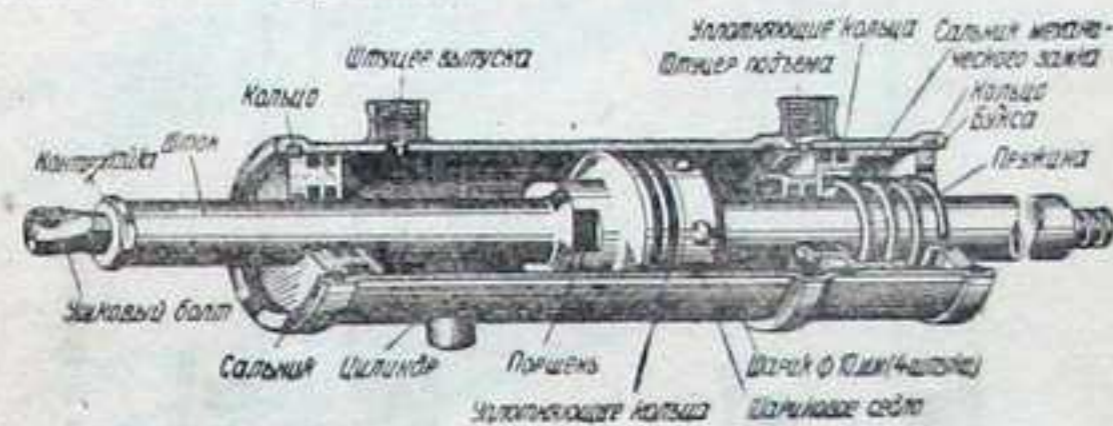
Фиг. 97. Подъемник закрылков.
