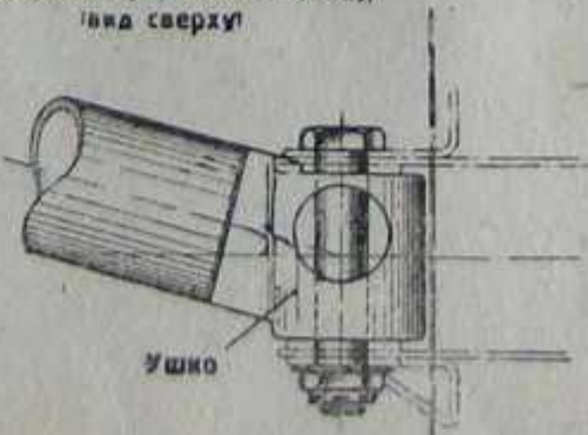
Фиг. 113. Узлы крепления моторной рамы и мотора.
