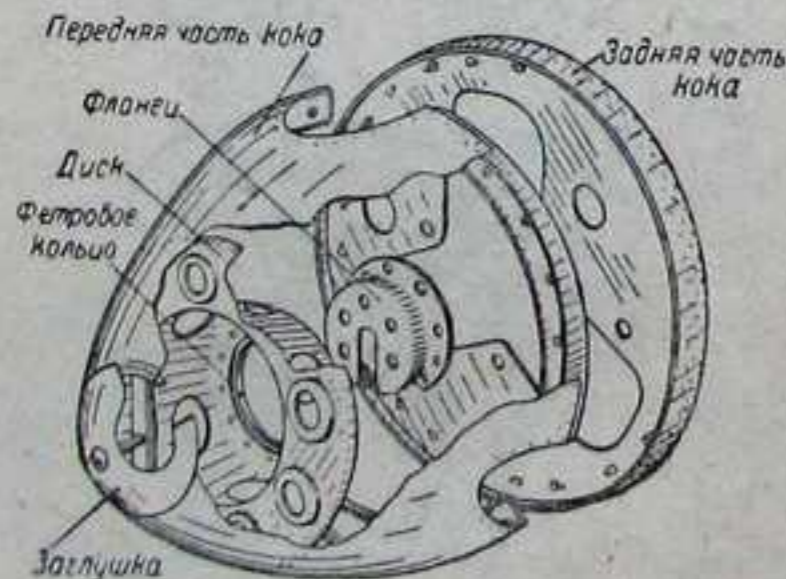
Фиг. 143. Кок винта.
