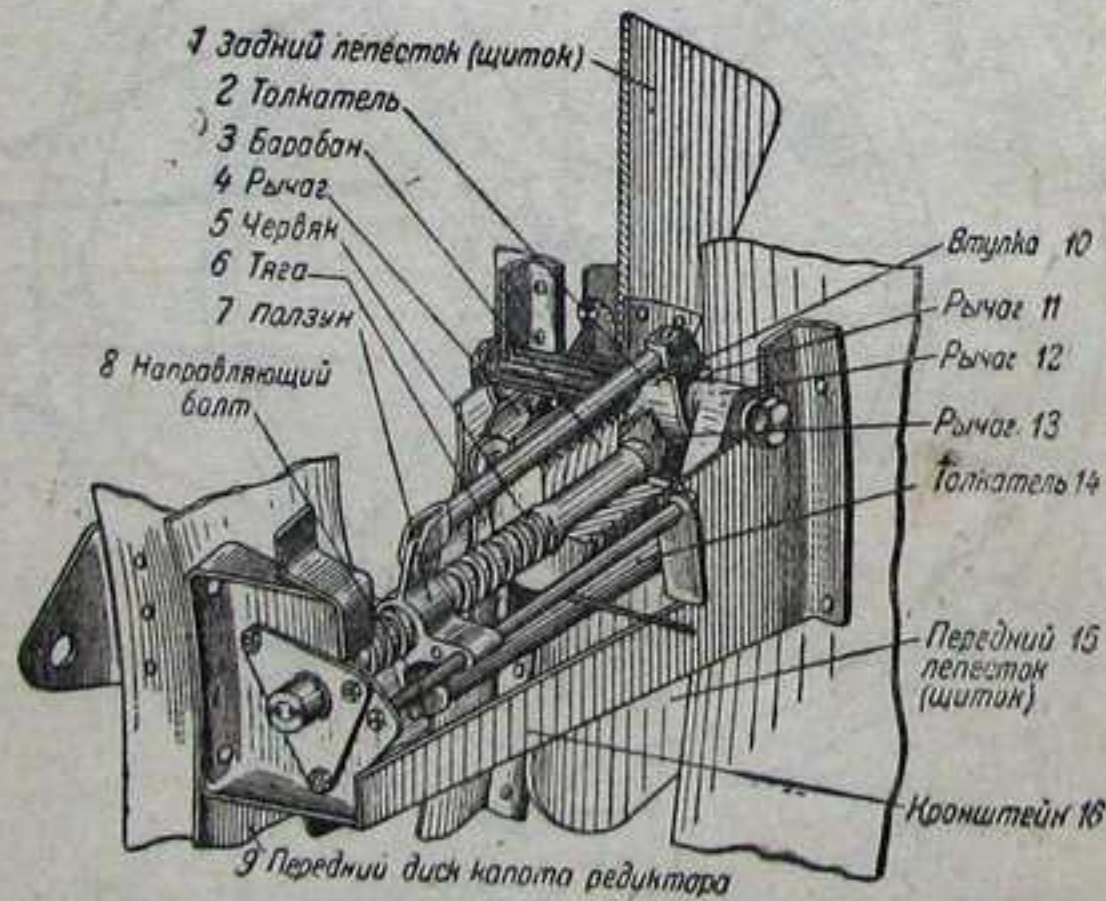
Фиг. 141. Механизм управления жалюзи.
