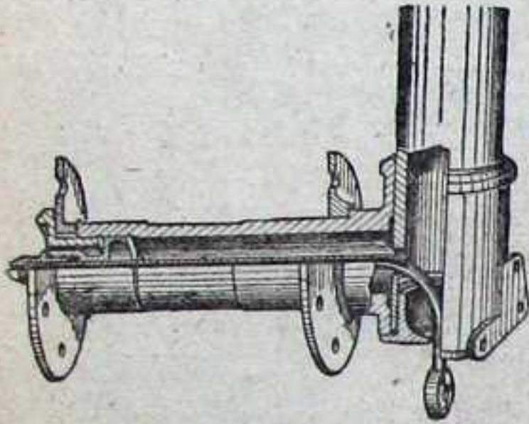
Фиг. 39. Полуось шасси.
