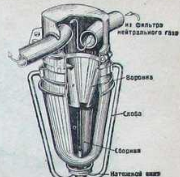
Фиг. 127. Бачок-сборник.
