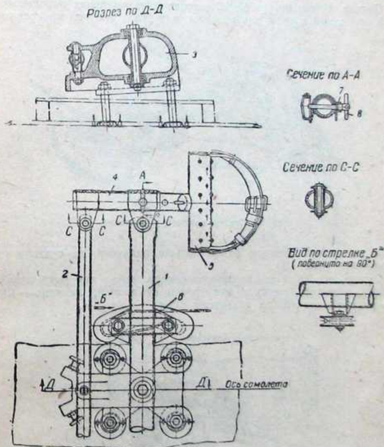
Фиг. 91. Педаль ножного управления.
