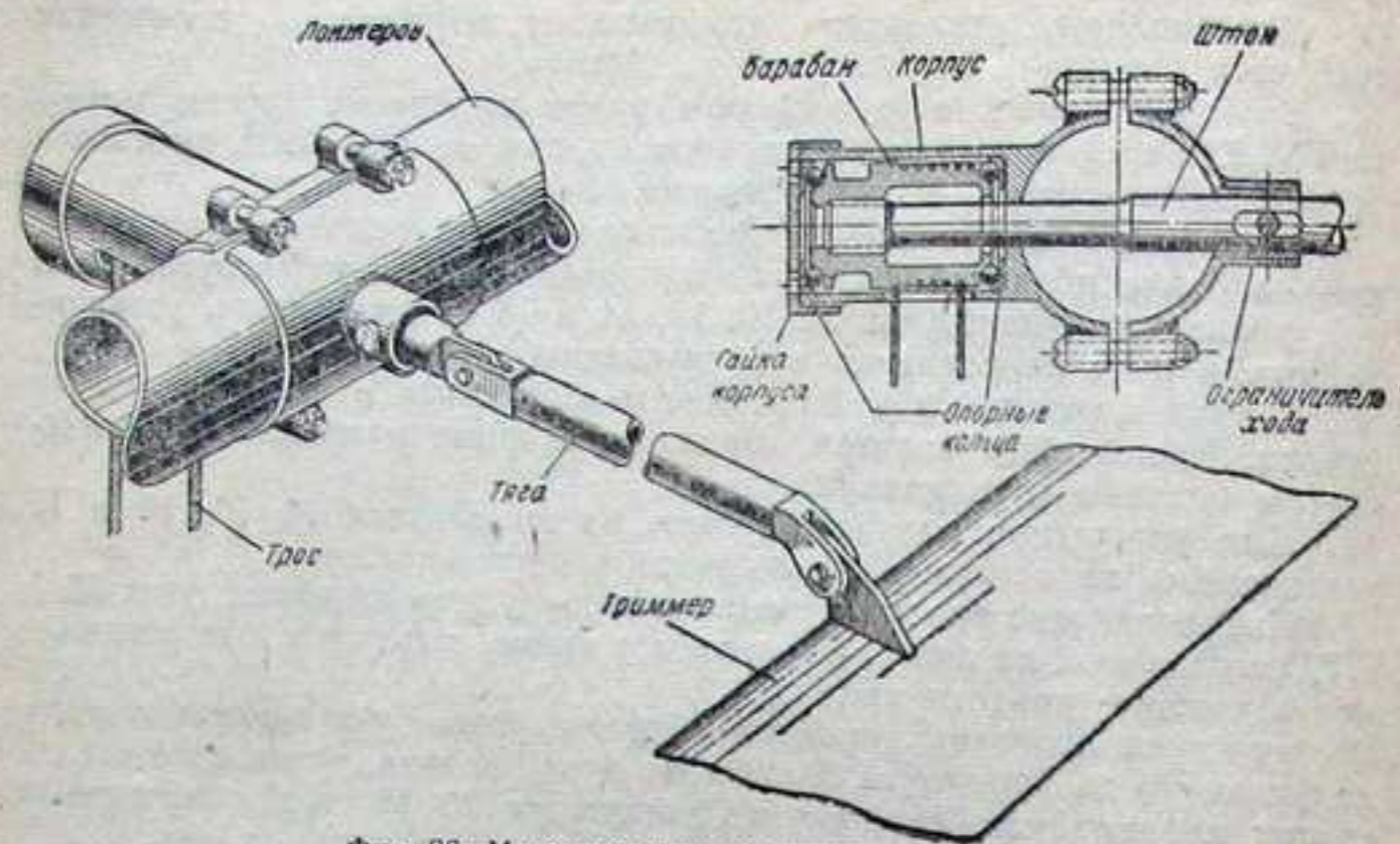
Фиг. 96. Механизм управления триммером.
