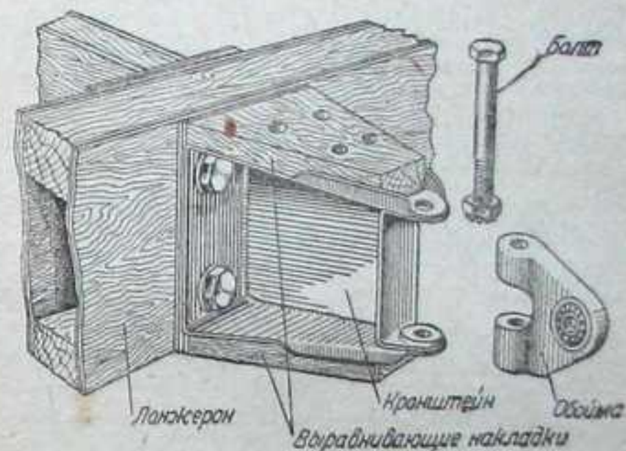
Фиг. 31. Кронштейн навески руля высоты.
