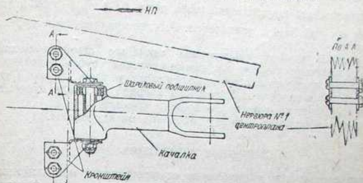
Фиг. 89. Качалка управления элеронами на нервюре № 1 центроплана.
