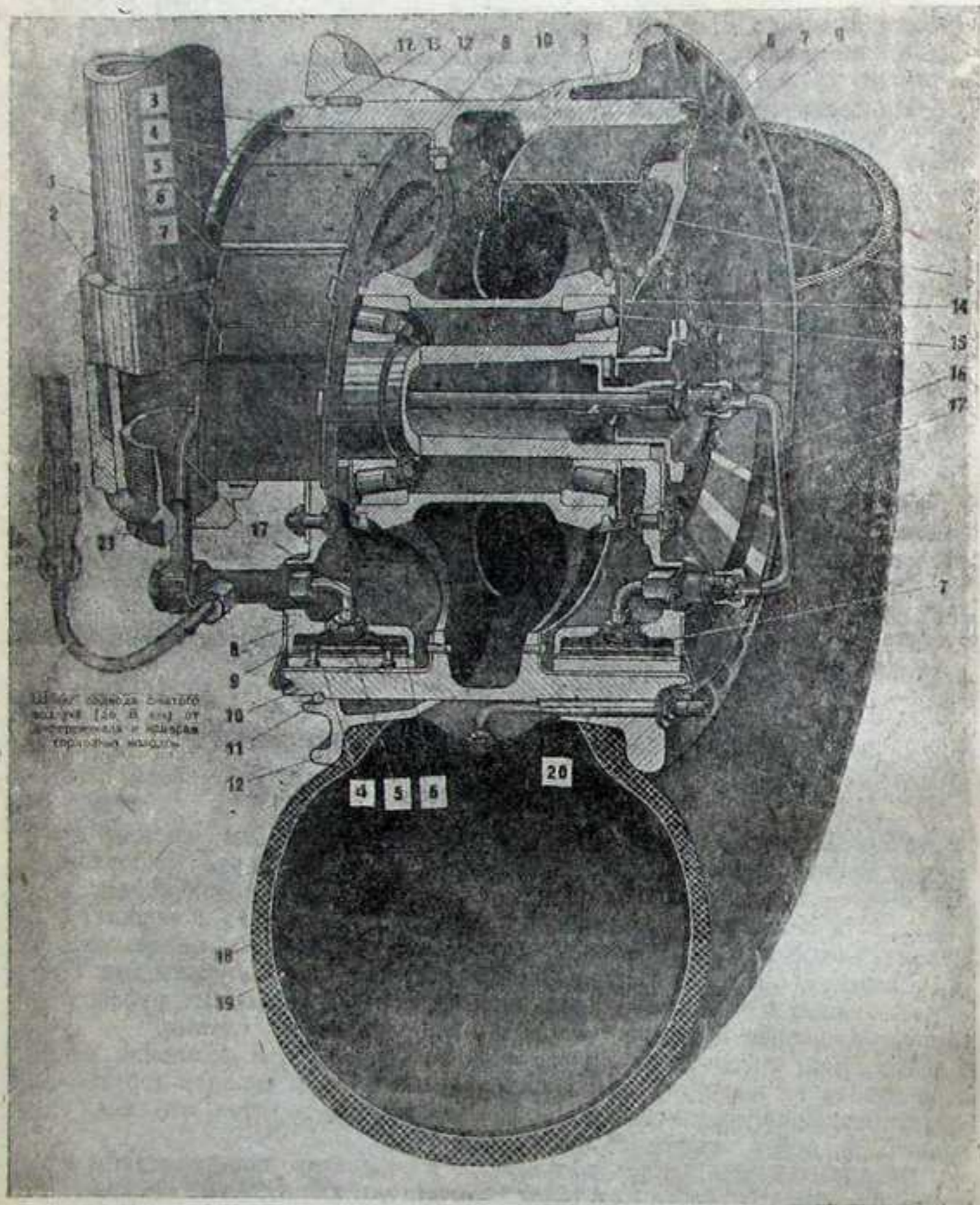
Фиг. 76. Колесо шасси.
