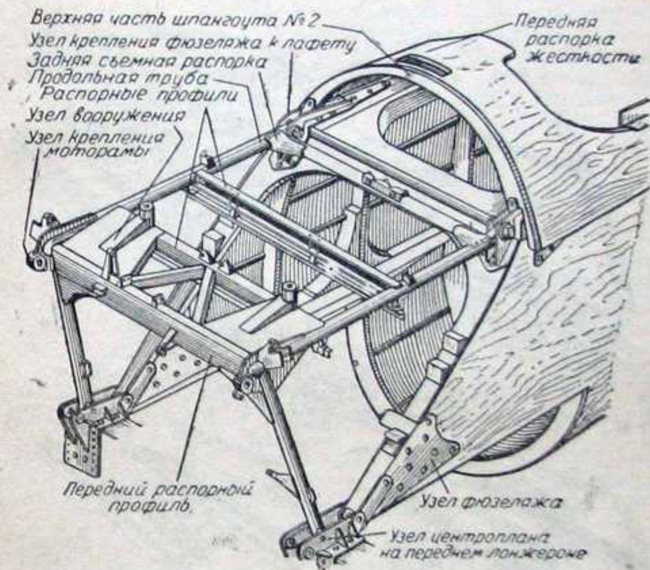
Фиг. 10. Лафет.
