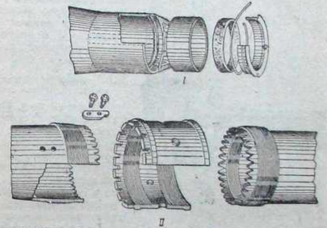
Фиг. 38. Детали соединения полови цилиндра амортизационной стойки.
