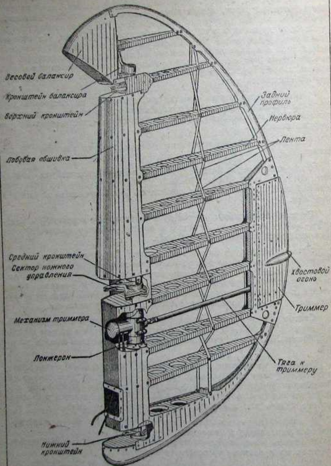
Фиг. 33. Руль направления.
