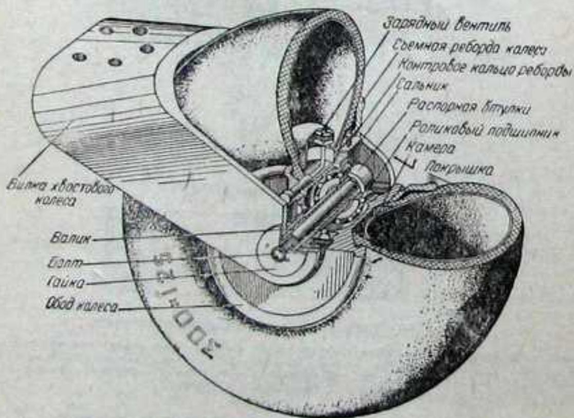
Фиг. 80. Хвостовое колесо.
