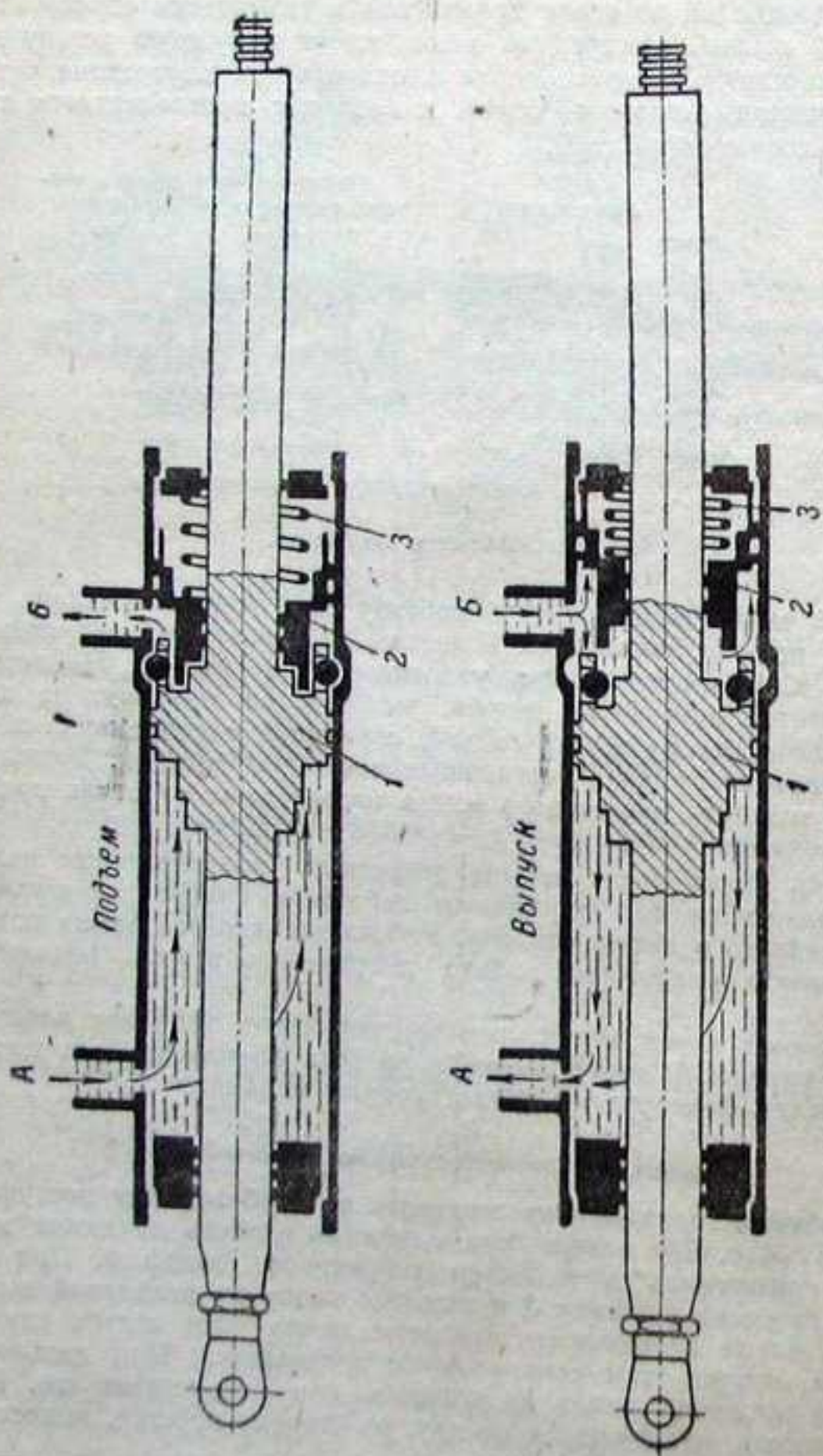
Фиг. 98. Принципиальная схема работы подъемника закрылков.
