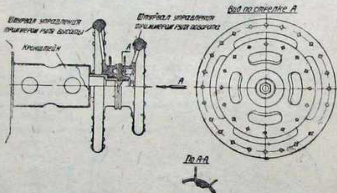
Фиг. 95. Штурвалы управления триммерами.
