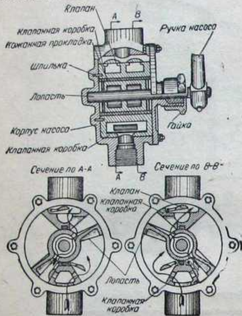
Фиг. 124. Схема работы альвейера.
