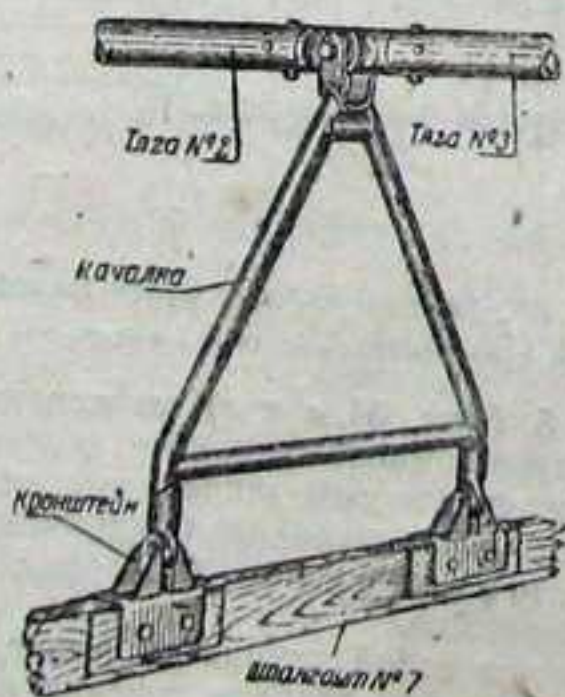
Фиг. 86. Качалка на шпангоуте № 7.
