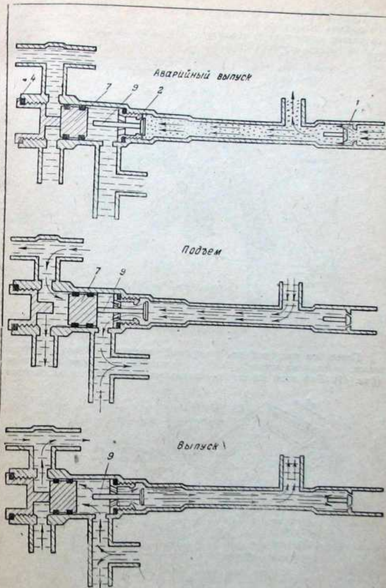
Фиг. 45. Принципиальная схема распределительной коробки подъемника шасси.
