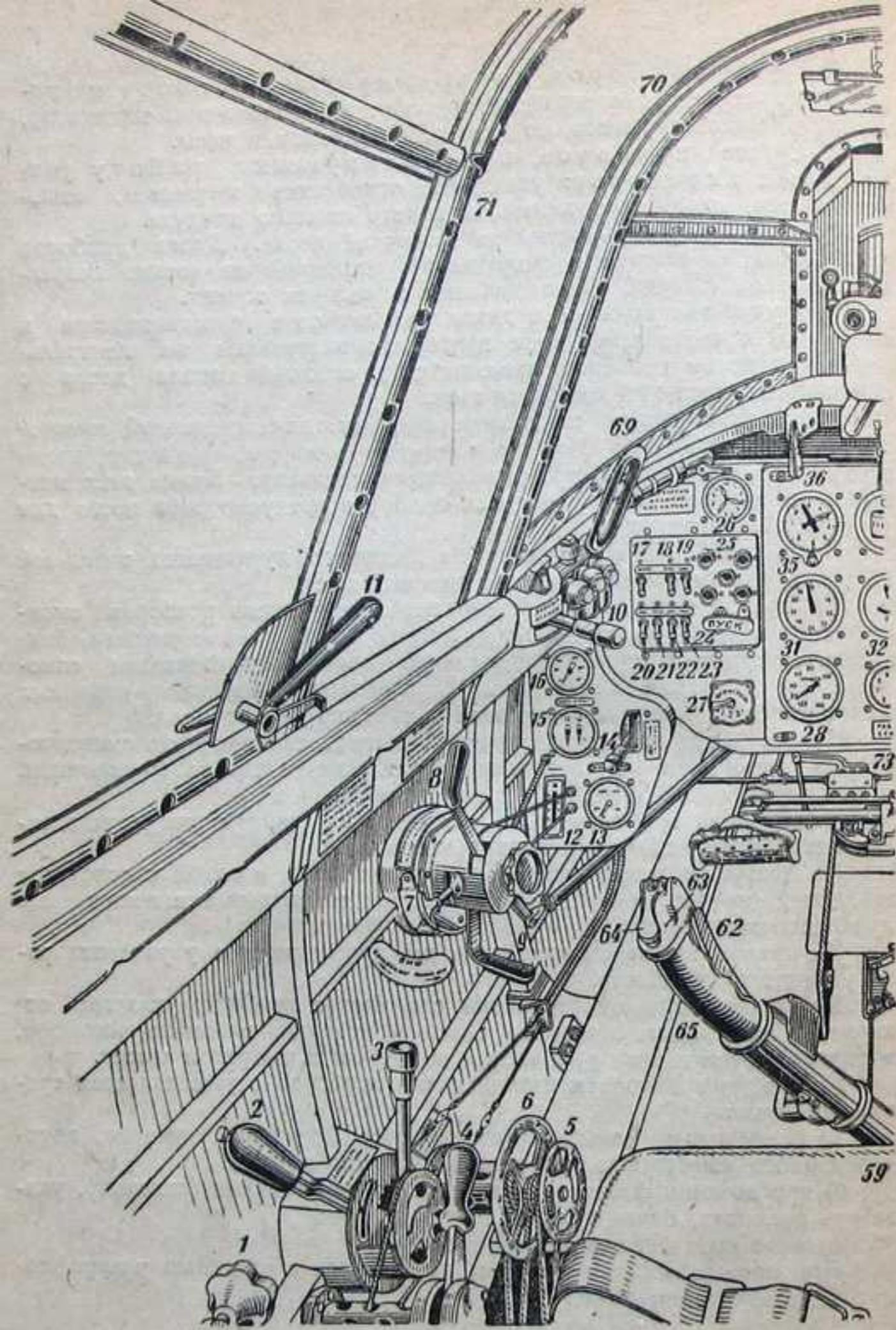
Фиг. 145. Кабина
