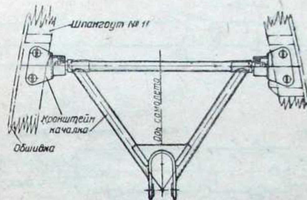
Фиг. 87. Качалки на шпангоутах № 9 и 11.
