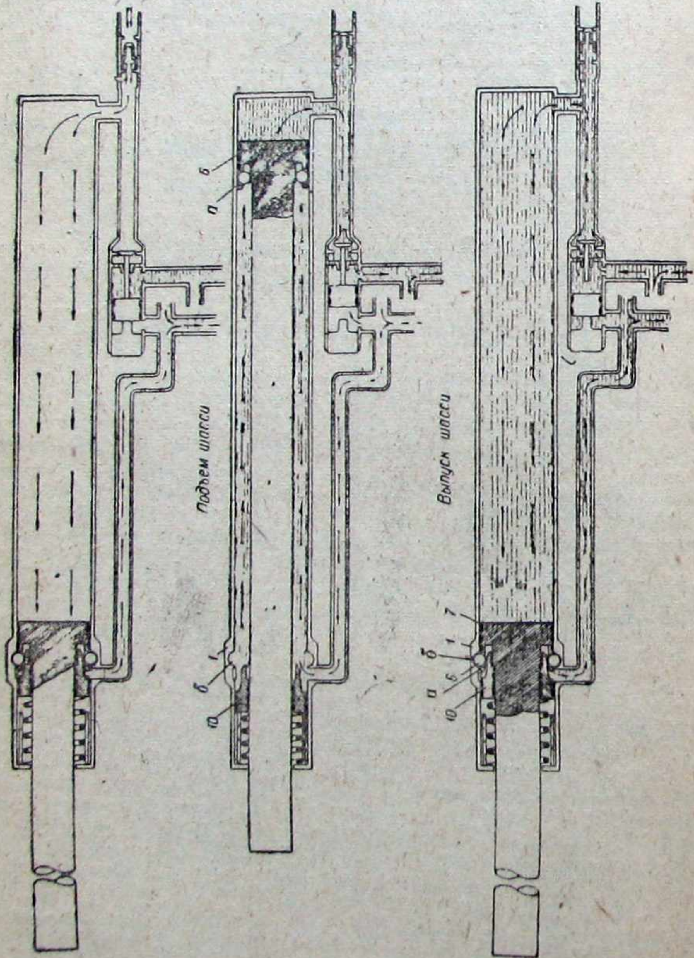
Фиг. 42. Принципиальная схема работы подъемника шасси.
