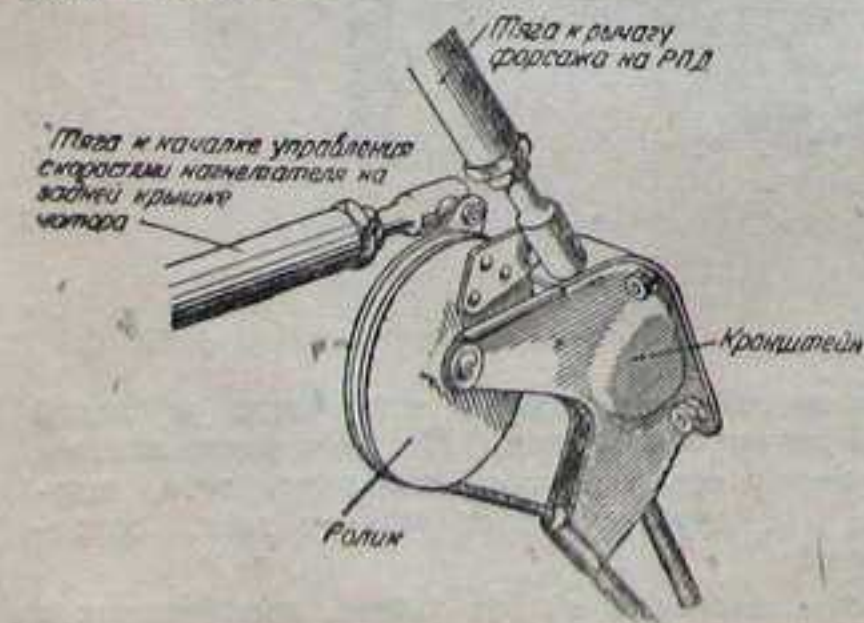
Фиг. 116. Ролик управления скоростями нагнетателя.
