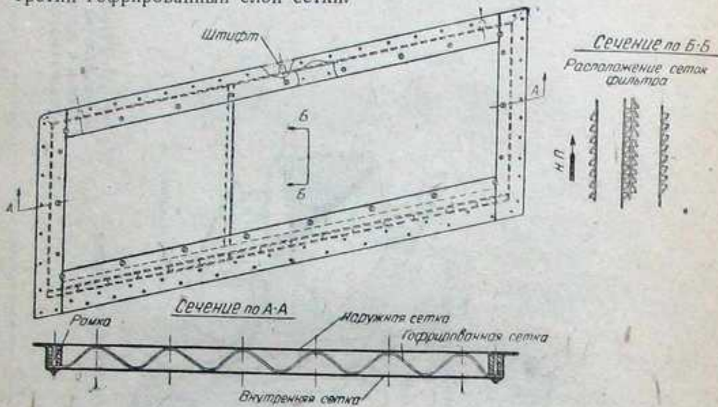
Фиг. 138. Сетчатый фильтр, установленный на всасывании.
