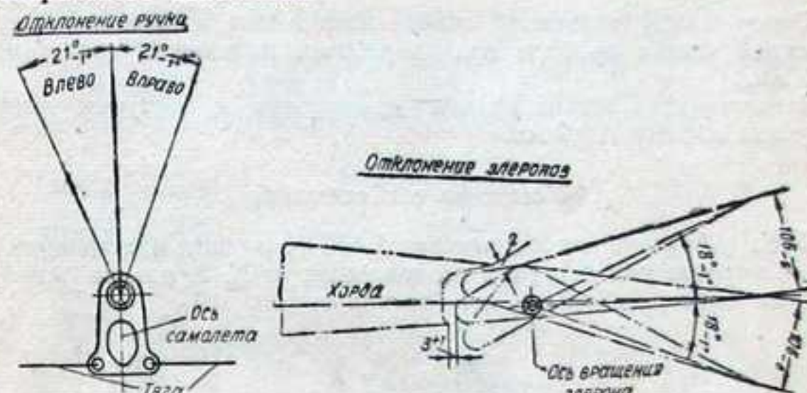
Фиг. 105. Регулировка управления элеронами.
