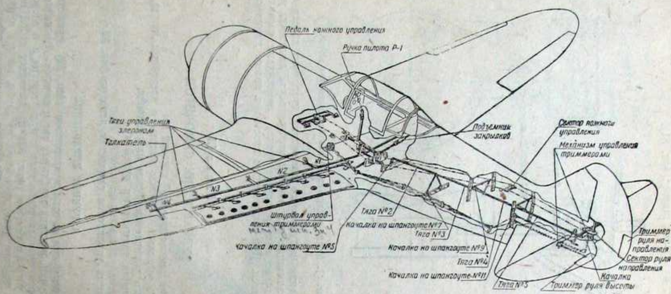
Фиг. 82. Управление самолетом.
