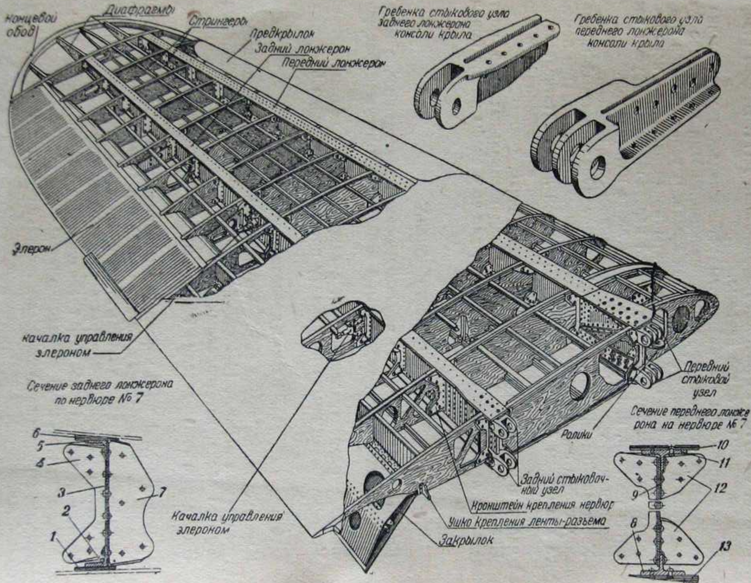
Фиг. 21. Консоль крыла.
