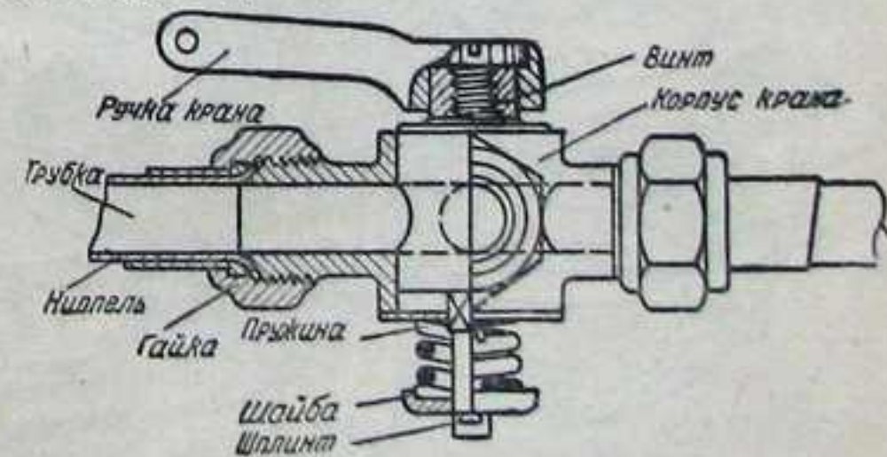
Фиг. 128. Перекрывной кран нейтрального газа.
