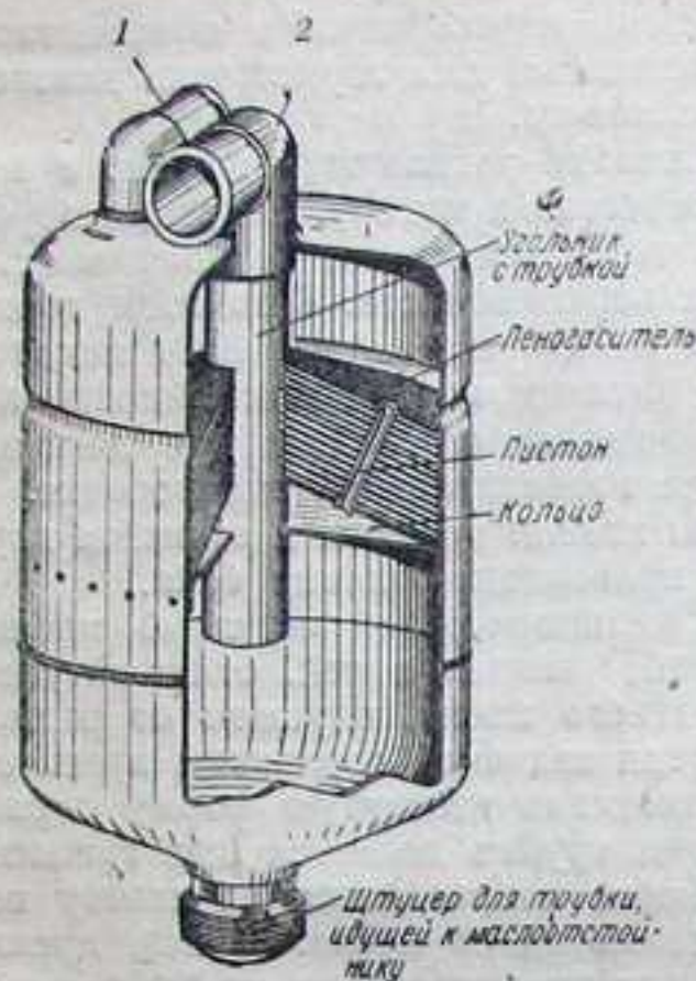
Фиг. 132. Дренажный бачок.
