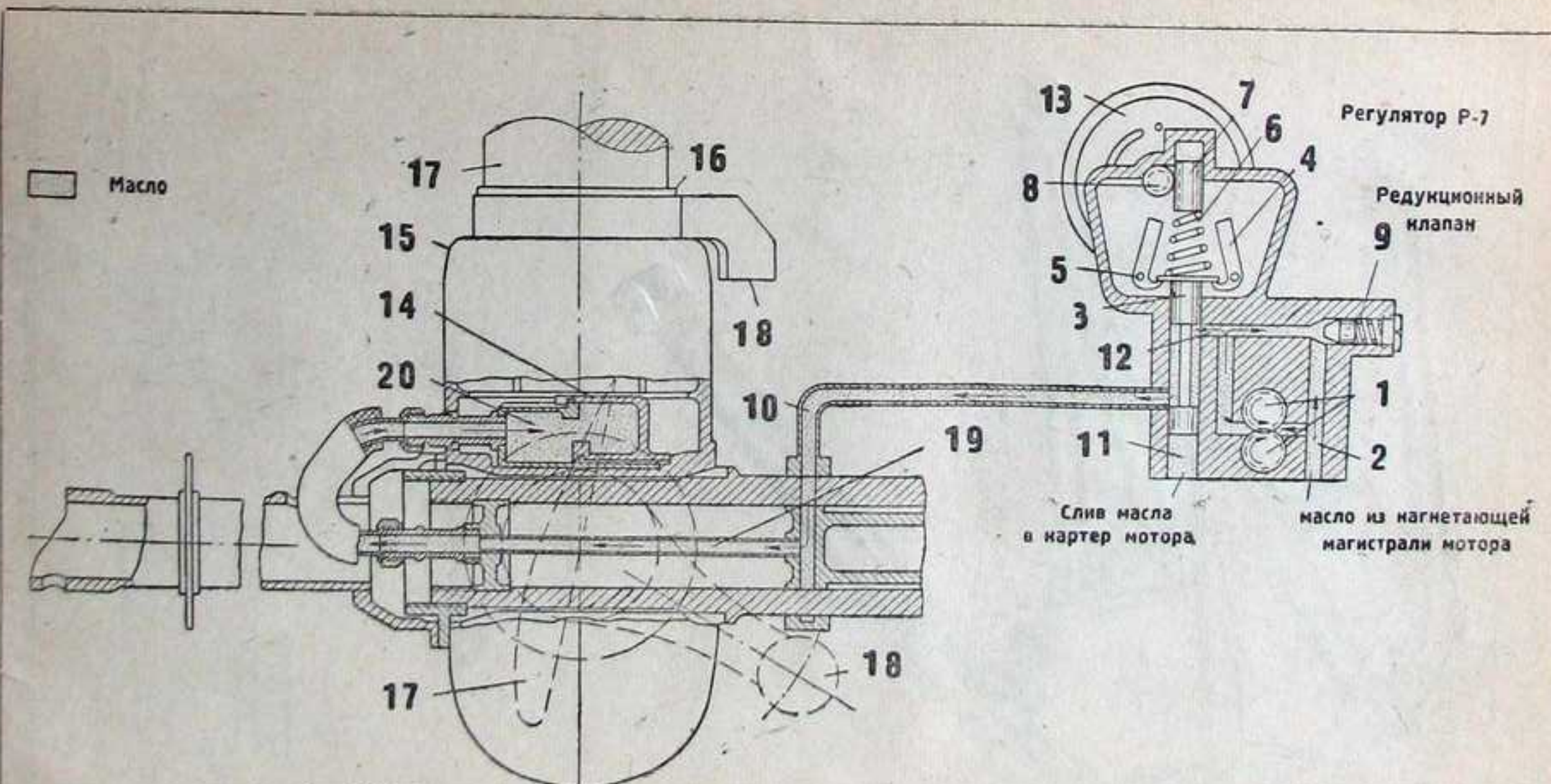
Фиг. 111б. Положение механизма переключения и регулятора винта при переводе на малый шаг.
