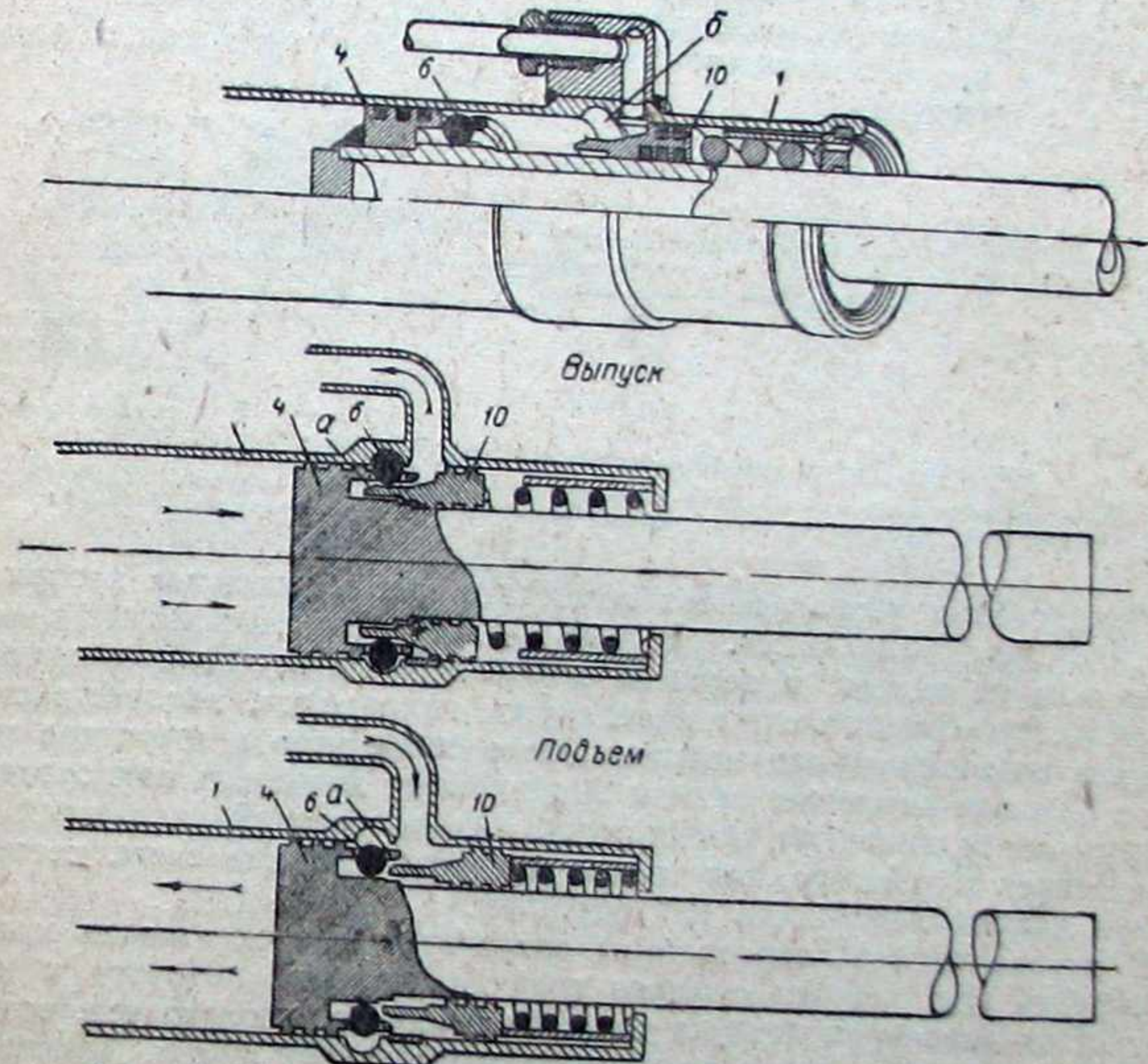
Фиг. 43. Шариковый замок подъемника и принцип его действия (обозначения те же, что и на фиг. 41 и 42).
