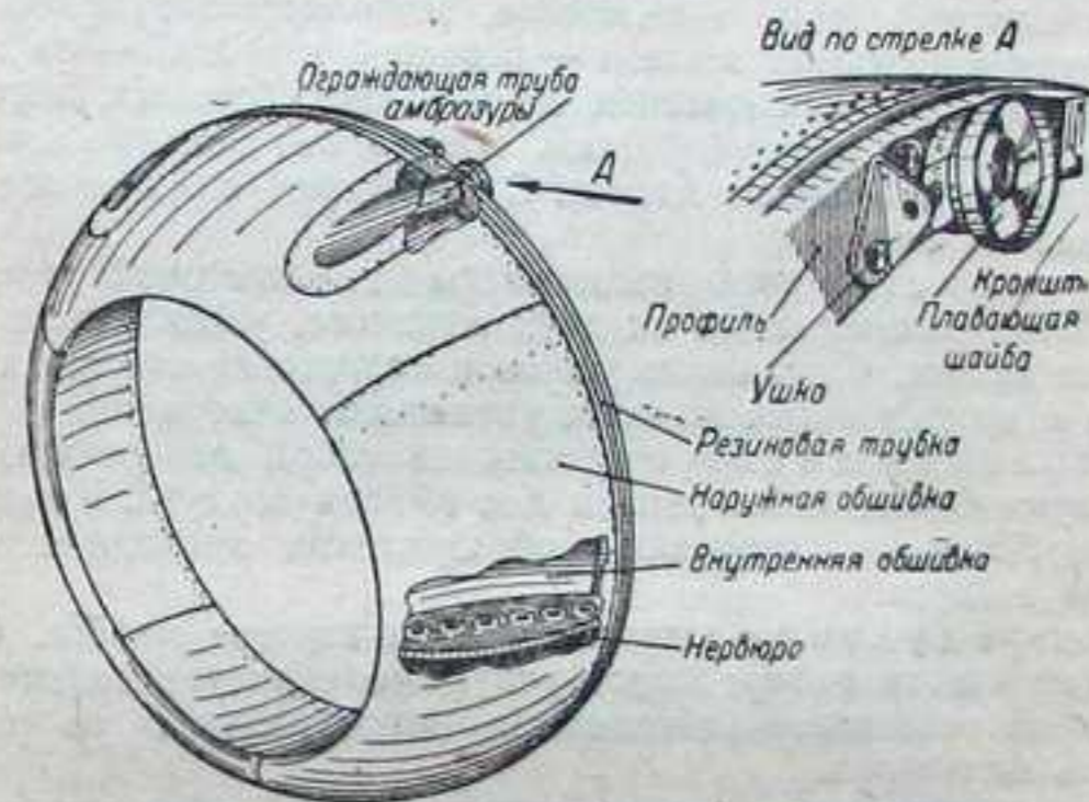
Фиг. 144. Переднее кольцо капота.
