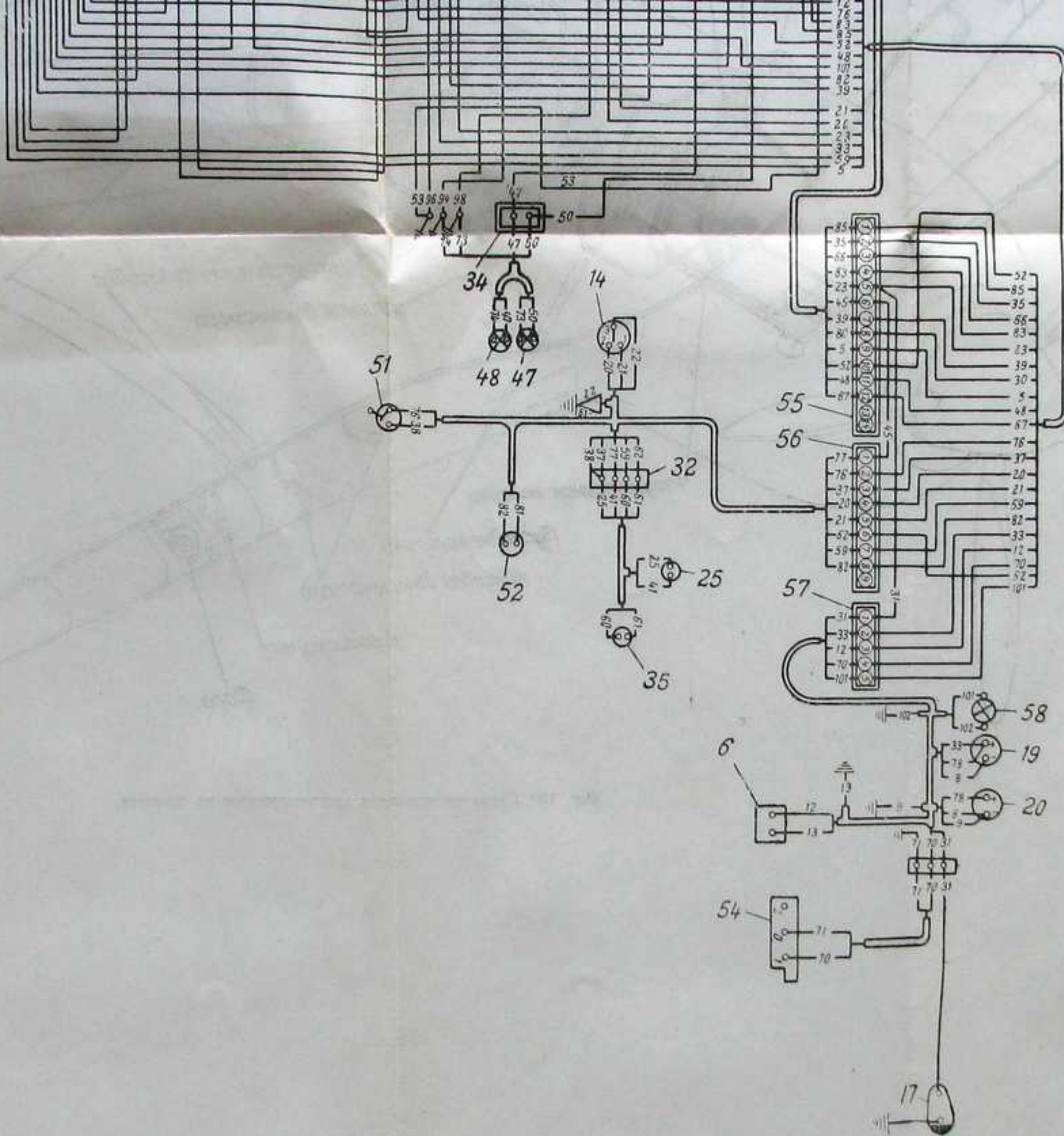
Фиг. 149. Полумонтажная схема электрооборудования.
