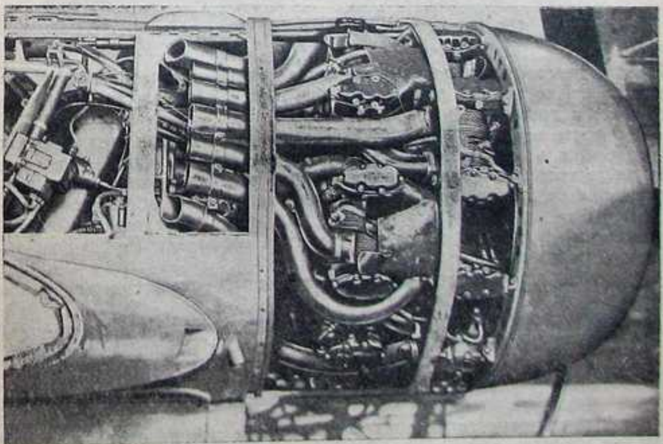
Фиг. 135. Выхлопные патрубки мотора. Правая группа.
