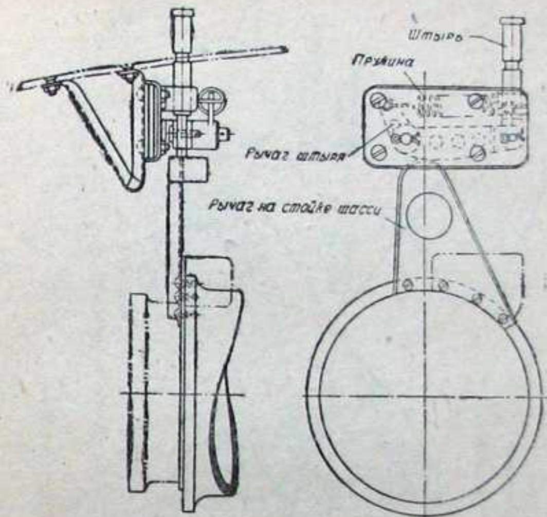
Фиг. 81. Механическая сигнализация положения шасси.
