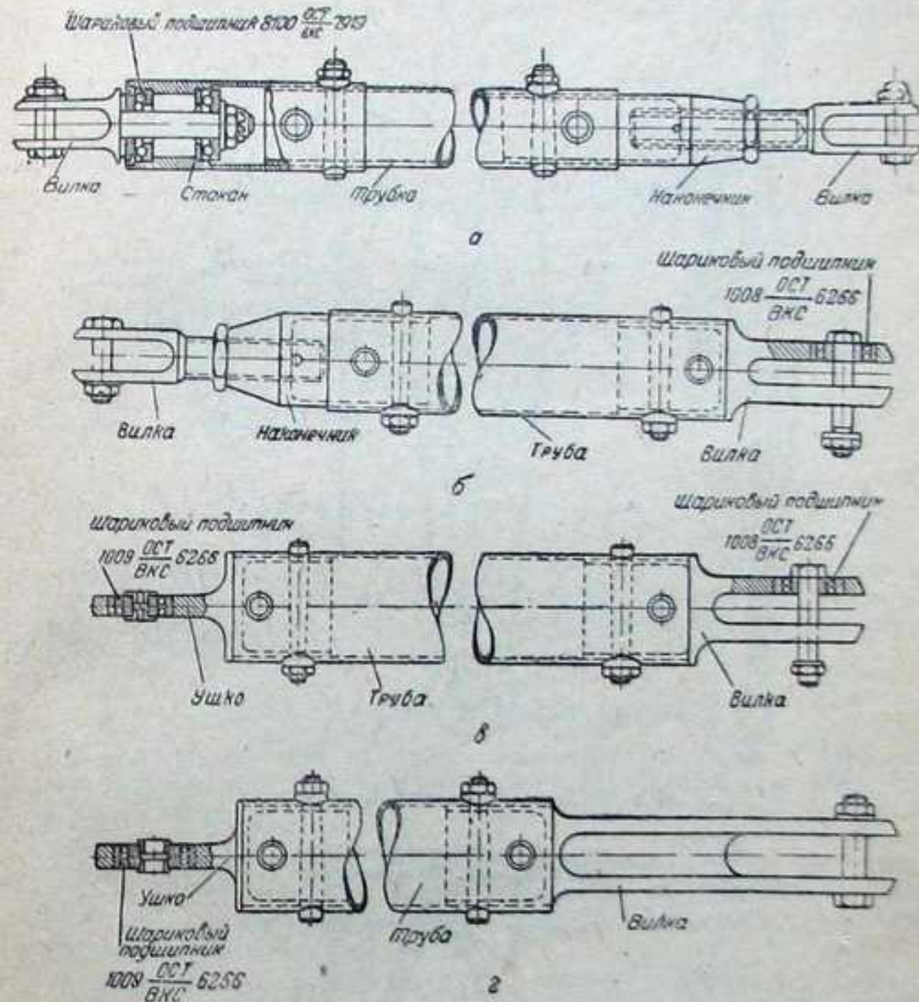
Фиг. 84. Тяги управления рулем высоты. а—тяга № 1; б—тяга № 2; в—тяги № 3 и 4; г—тяга № 5.
