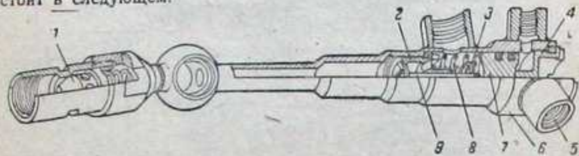
Фиг. 44. Распределительная коробка подъемника шасси.
