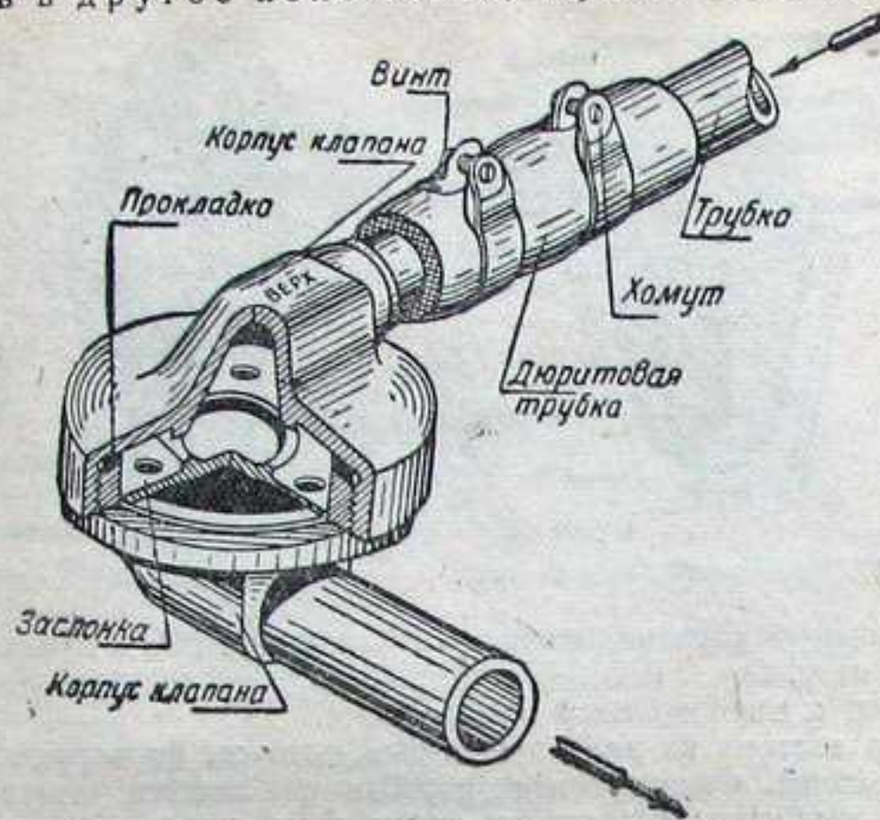
Фиг. 129. Обратный клапан нейтрального газа.
