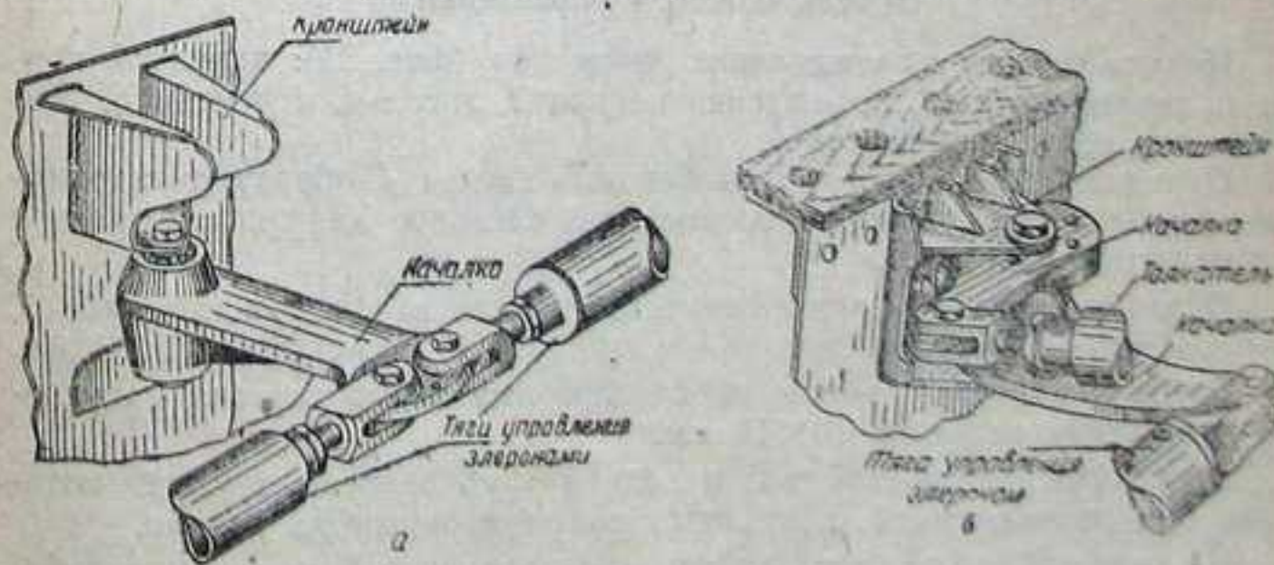
Фиг. 90. Качалка управления элеронами.
