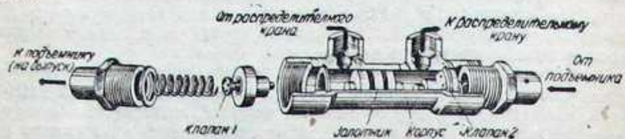
Фиг. 69. Двухсторонний клапан подъемника закрылков (такой же клапан имеется у подъемника хвостового колеса).
