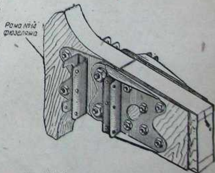
Фиг. 29. Стыковой узел заднего лонжерона стабилизатора.
