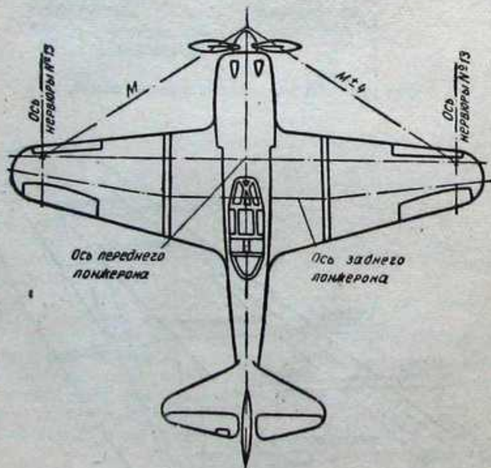
Фиг. 104. Проверка стреловидности крыла.
