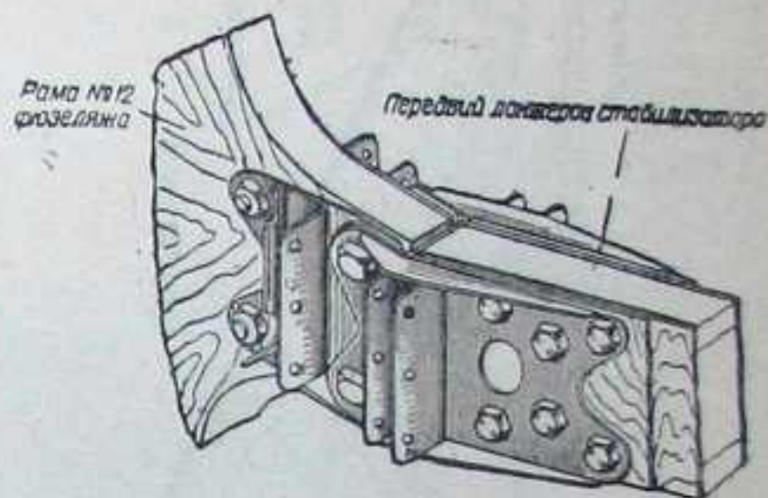
Фиг. 28. Стыковой узел переднего лонжерона стабилизатора.
