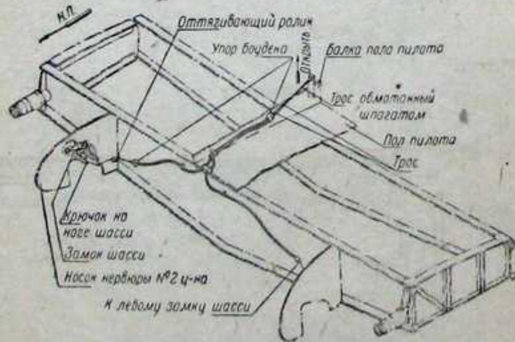
Фиг. 47. Схема механического закрывания замков шасси.
