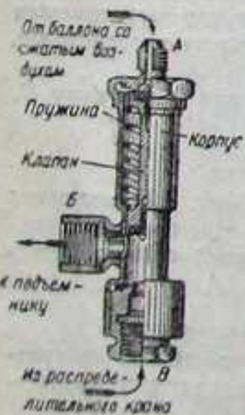
Фиг. 71. Аварийный воздушный клапан.
