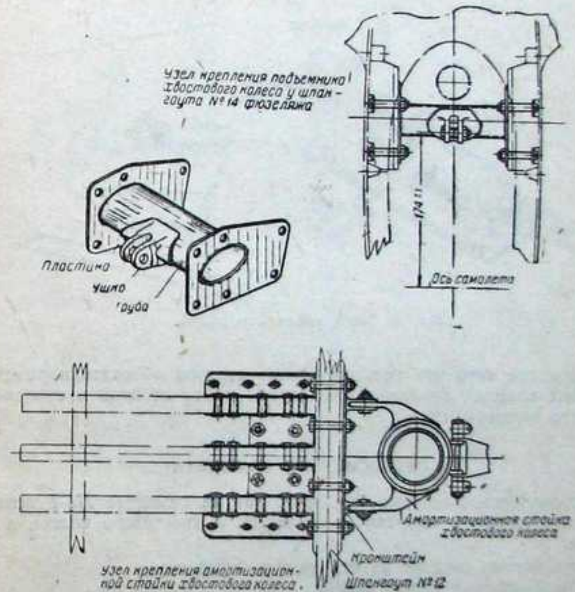
Фиг. 55. Узлы крепления подъемника хвостового колеса.
