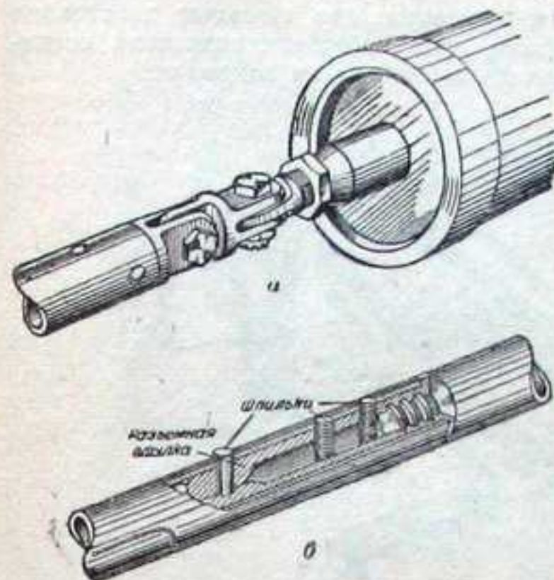
Фиг. 99. Детали проводки управления закрылками.
