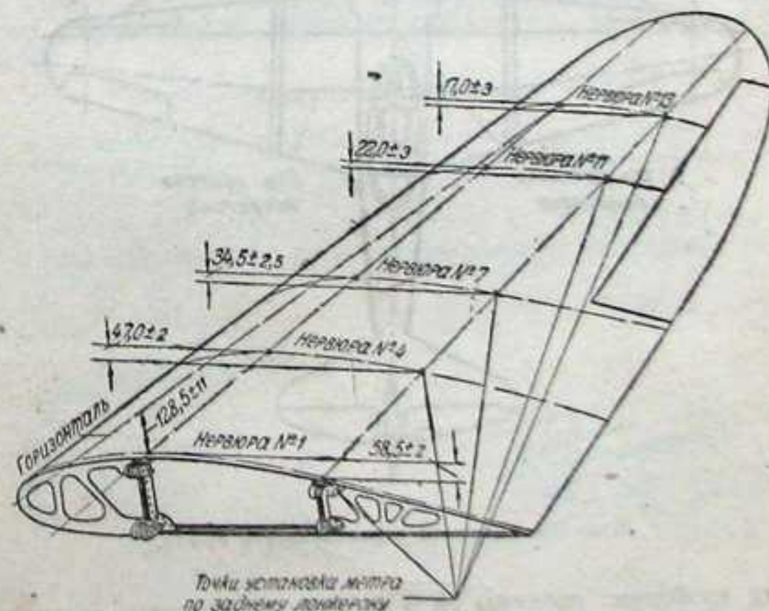
Фиг. 103. Регулировка крыла.
