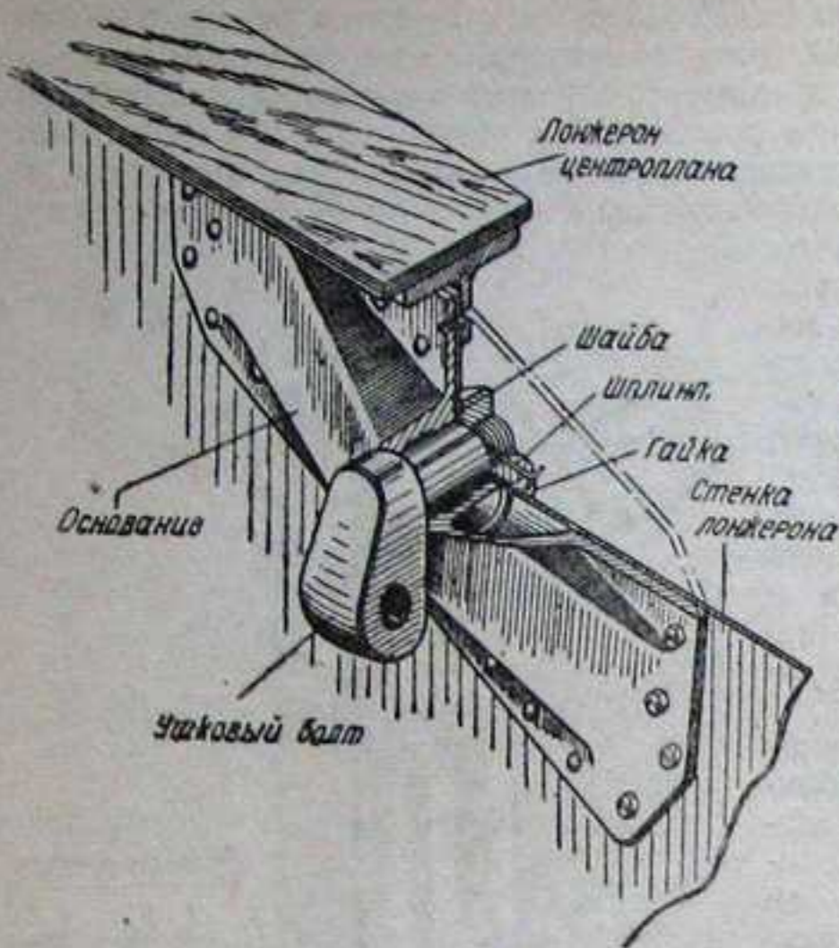
Фиг. 18. Узел крепления подъемника шасси.
