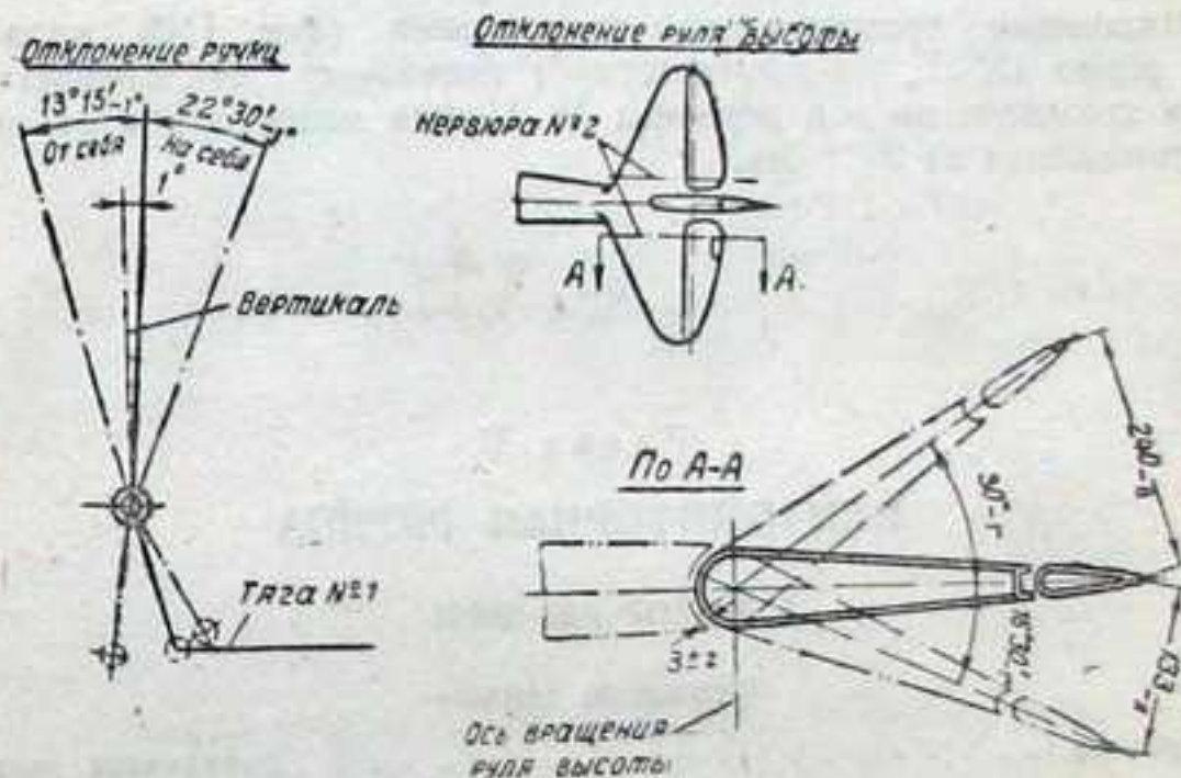
Фиг. 109. Регулировка управления рулем высоты.
