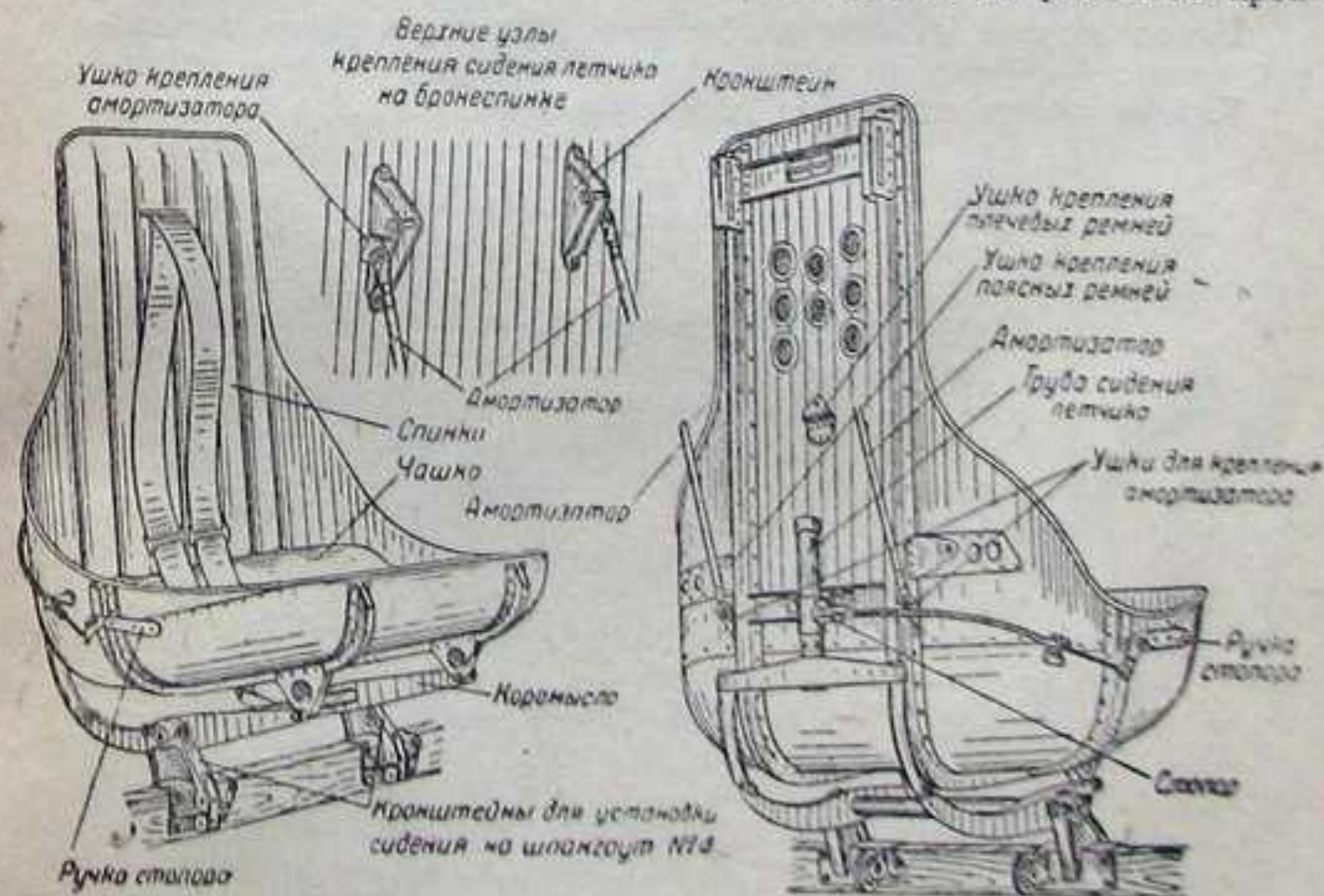
Фиг. 153. Сиденье пилота.
