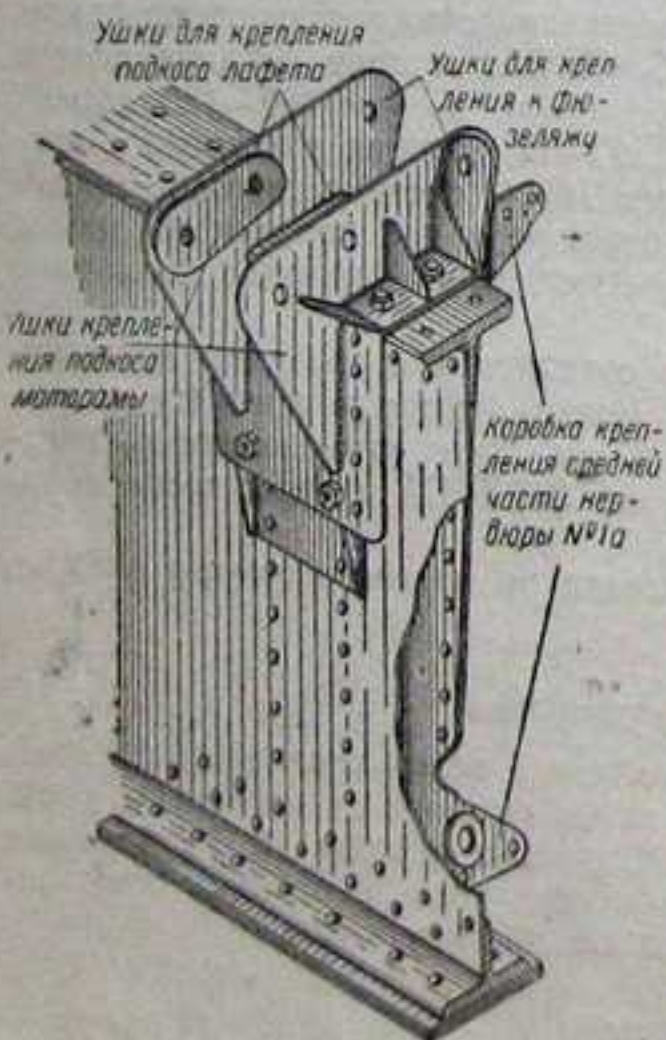
Фиг. 16. Передний узел крепления центроплана к фюзеляжу.
