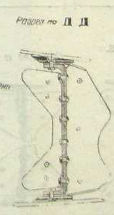
Фиг. 23. Задний лонжерон консоли крыла.
