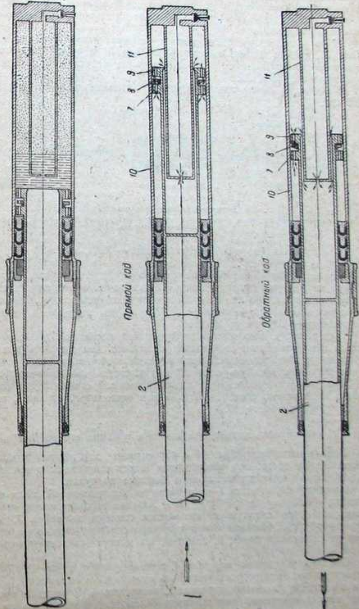
Фиг. 40. Схема работы амортизатора шасси (обозначения те же, что и на фиг. 37).
