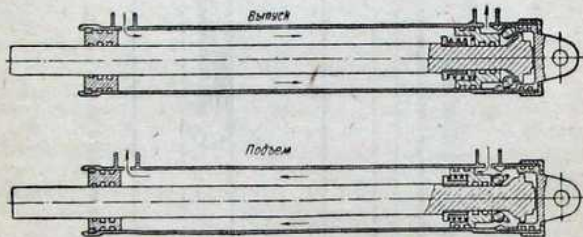
Фиг. 54. Принципиальная схема работы подъемника.
