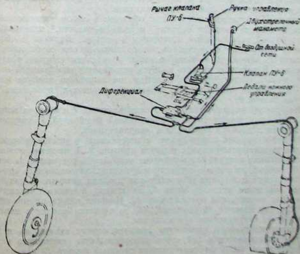
Фиг. 77. Схема управления тормозами.
