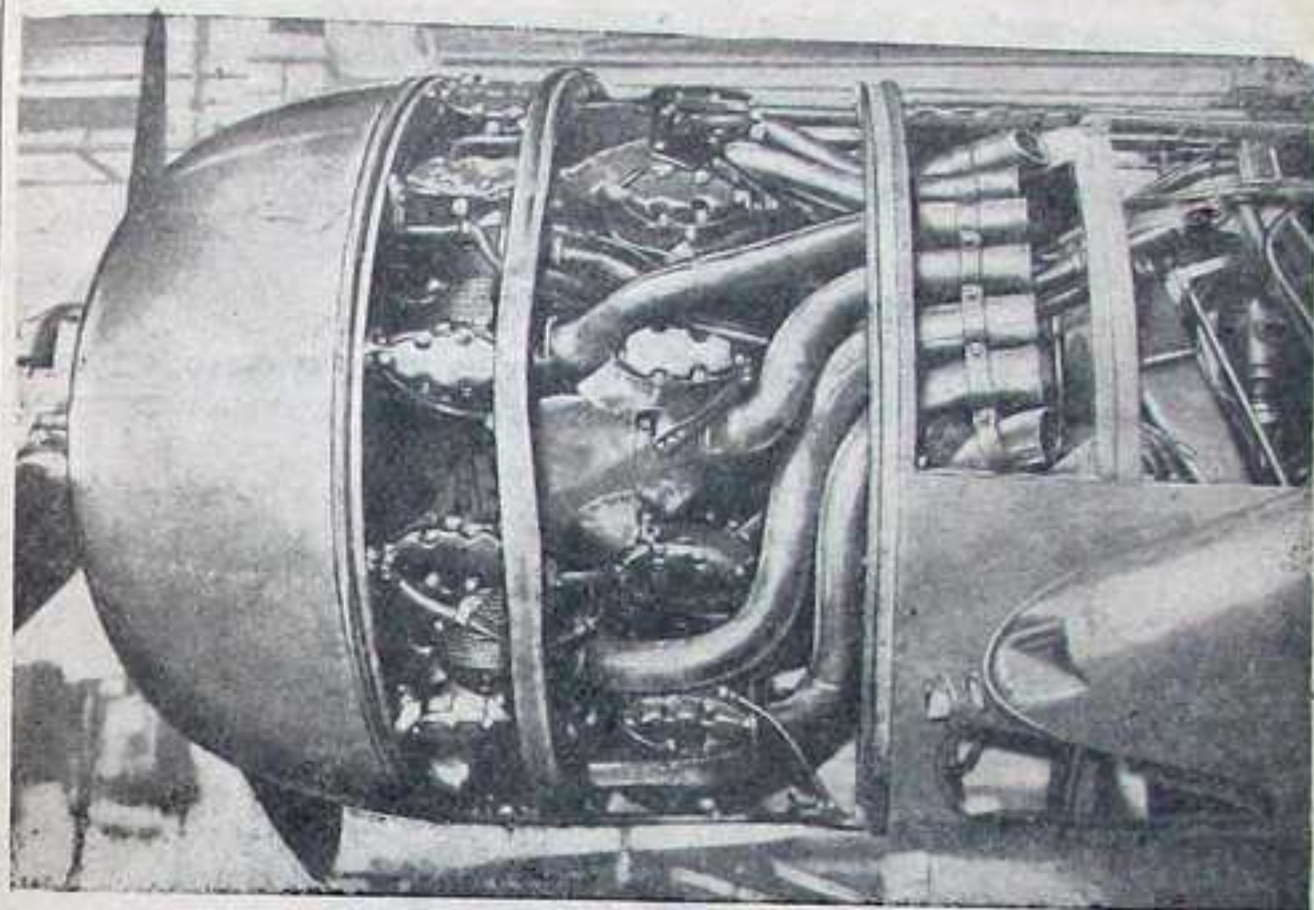
Фиг. 134. Выхлопные патрубки мотора. Левая группа.
