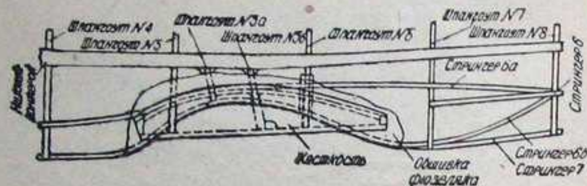
Фиг. 6. Нижняя часть фюзеляжа в месте установки туннеля маслорадиатора.
