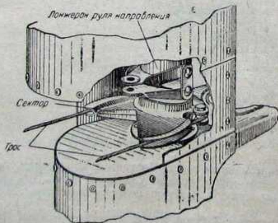
Фиг. 93. Сектор на руле направления.
