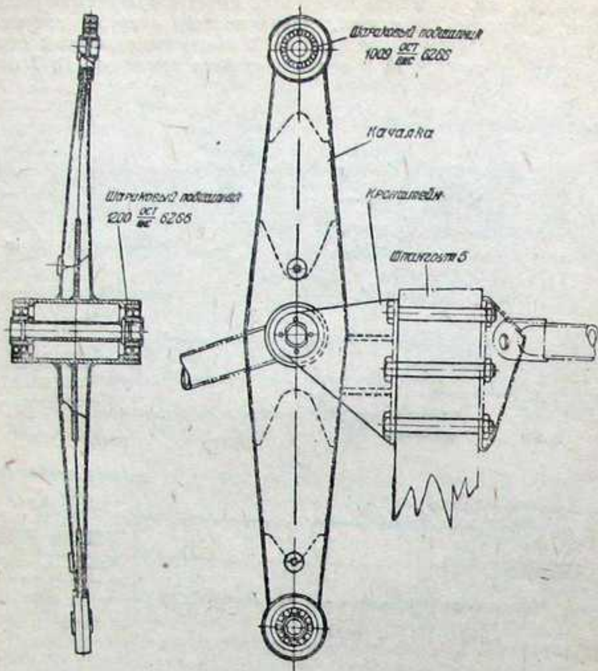
Фиг. 85. Качалка на шпангоуте № 5.
