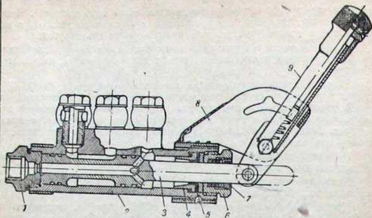
Фиг. 62. Распределительный кран закрылков (обозначения те же, что и на фиг. 61).
