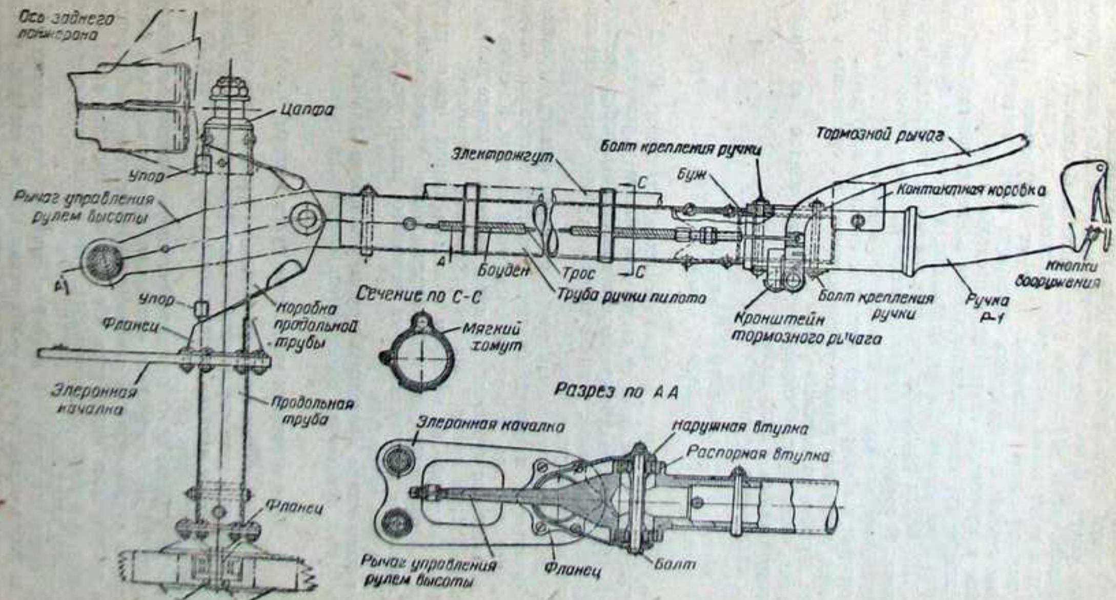
Фиг. 83. Ручка управления.
