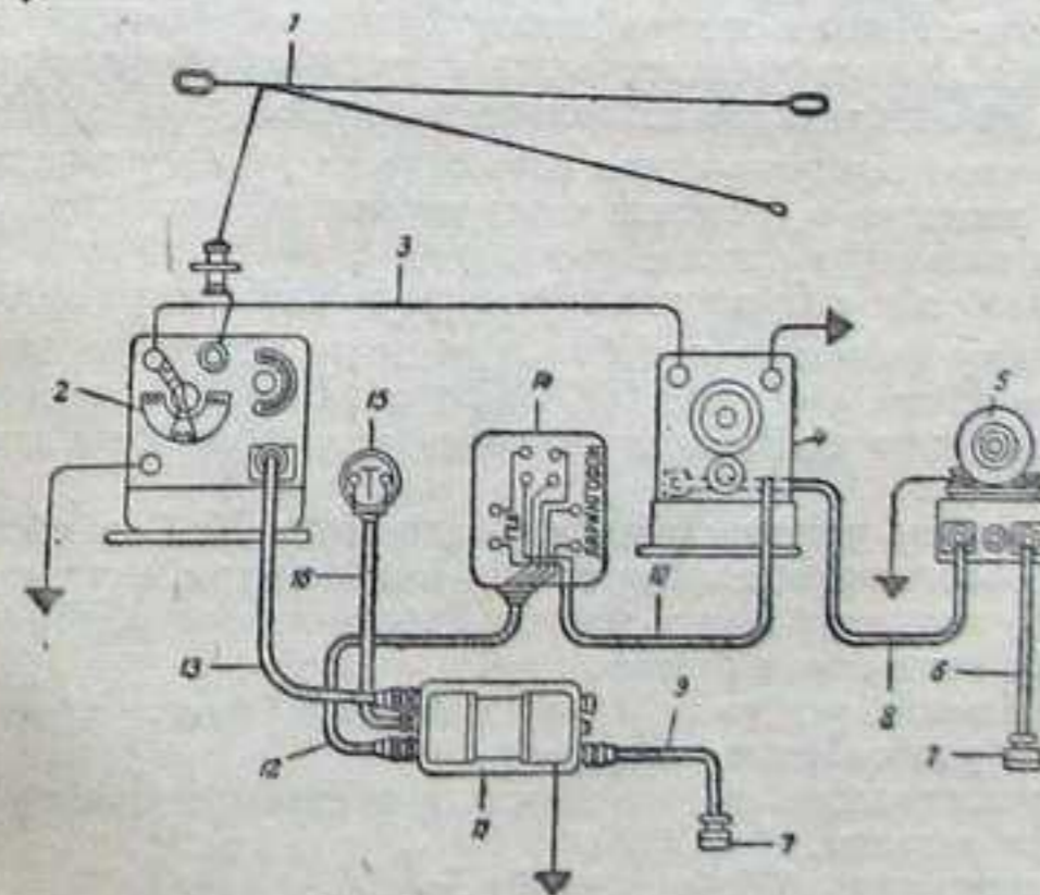
Фиг. 152. Схема установки радиостанции.
