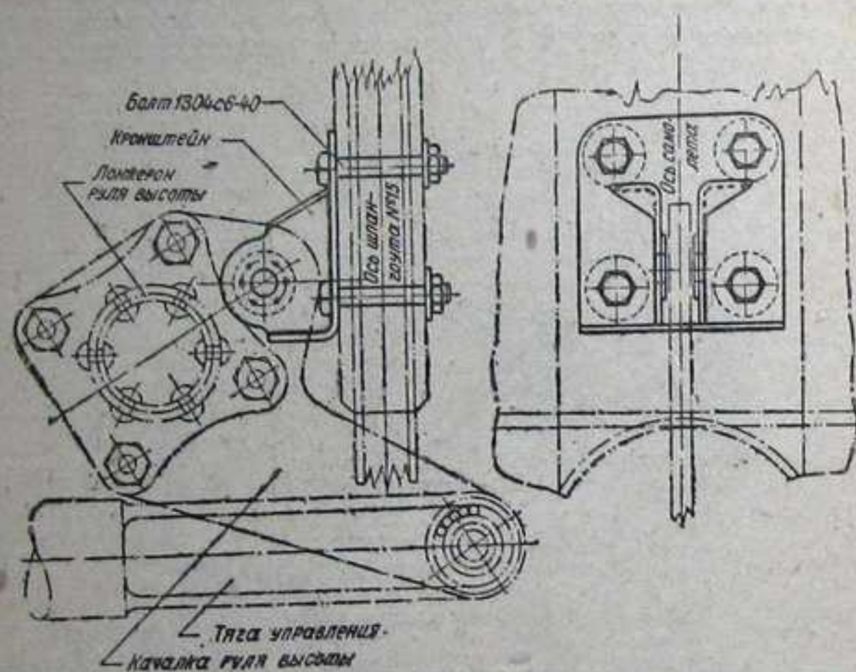
Фиг. 32. Качалка руля высоты.
